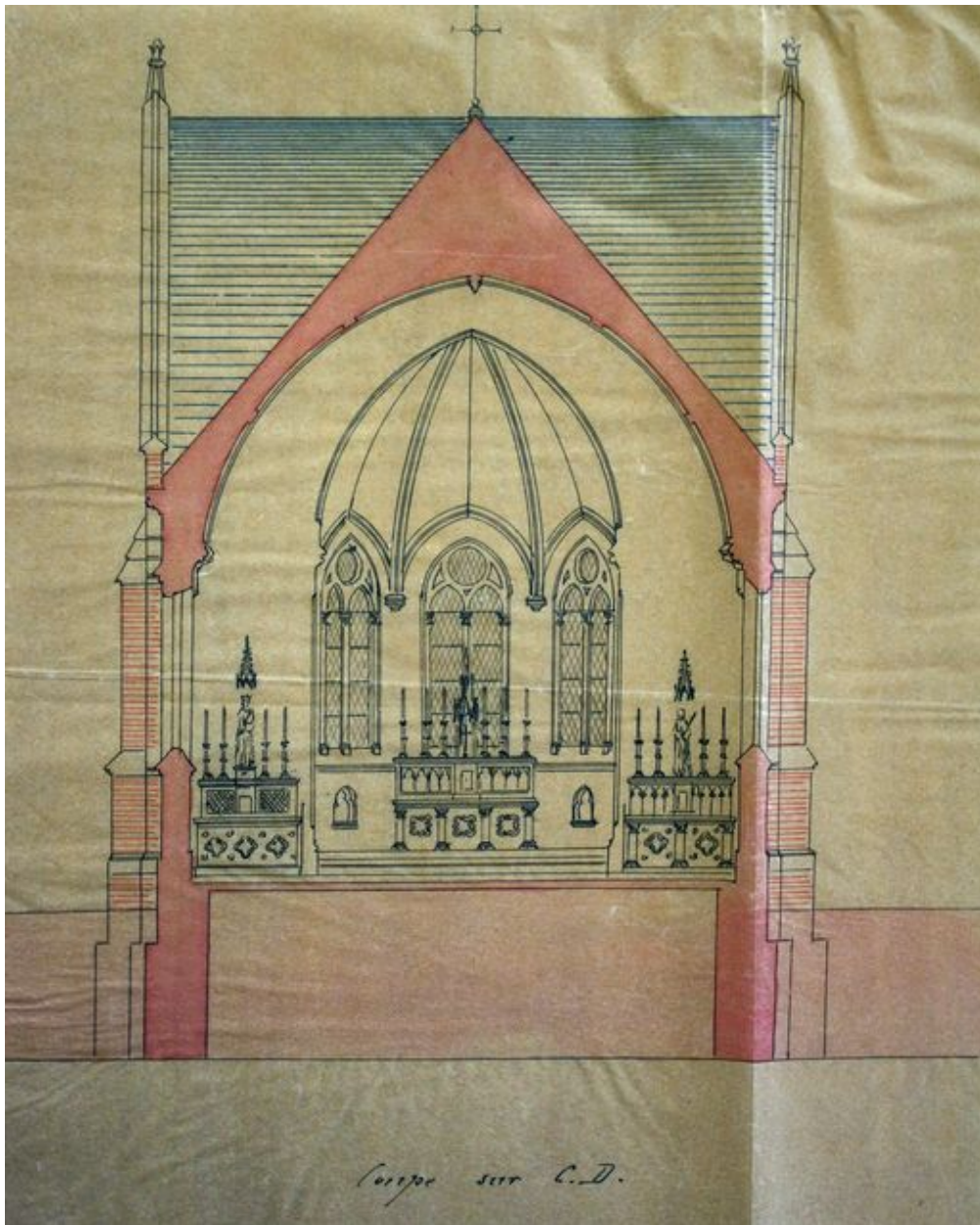
Coupe transversale de la nouvelle église, par Herbault (architecte), 1866 (AD Somme ; 99 O 3775).
