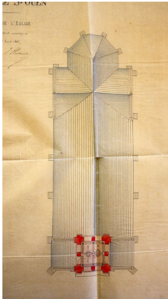
Plan des toitures de la nouvelle église, par Herbault (architecte), 1866 (AD Somme ; 99 O 3775).
