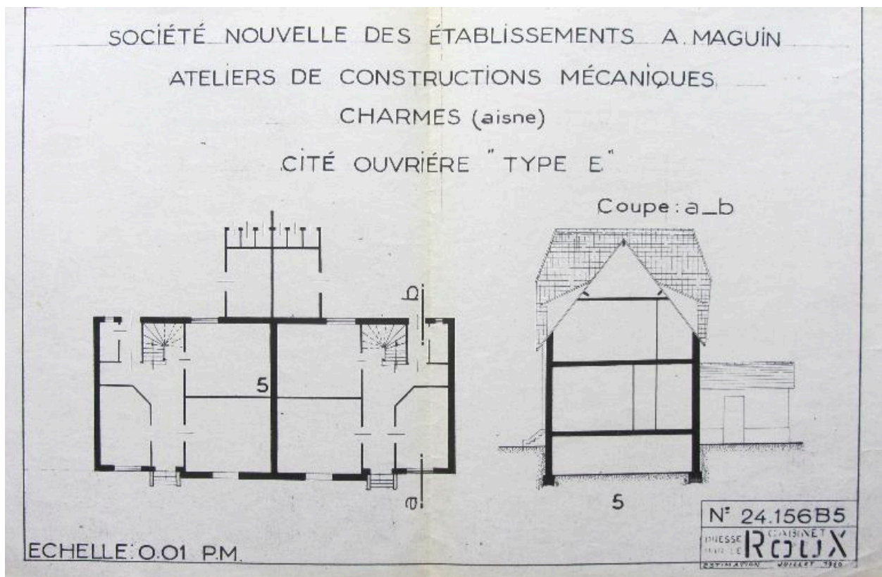
Cité ouvrière, type E. Plan et coupe. Cabinet Roux, juillet 1960 (Archives privées de l'entreprise).
