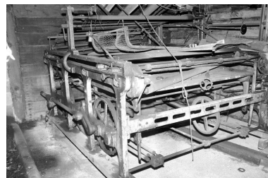
Plieuse. La plaque porte la mention : (IRION-VOSSELER) Scweningen et Rogo (Mulhouse), sans date Phot. Benoît Dufournier IVR22_19888000095Z
