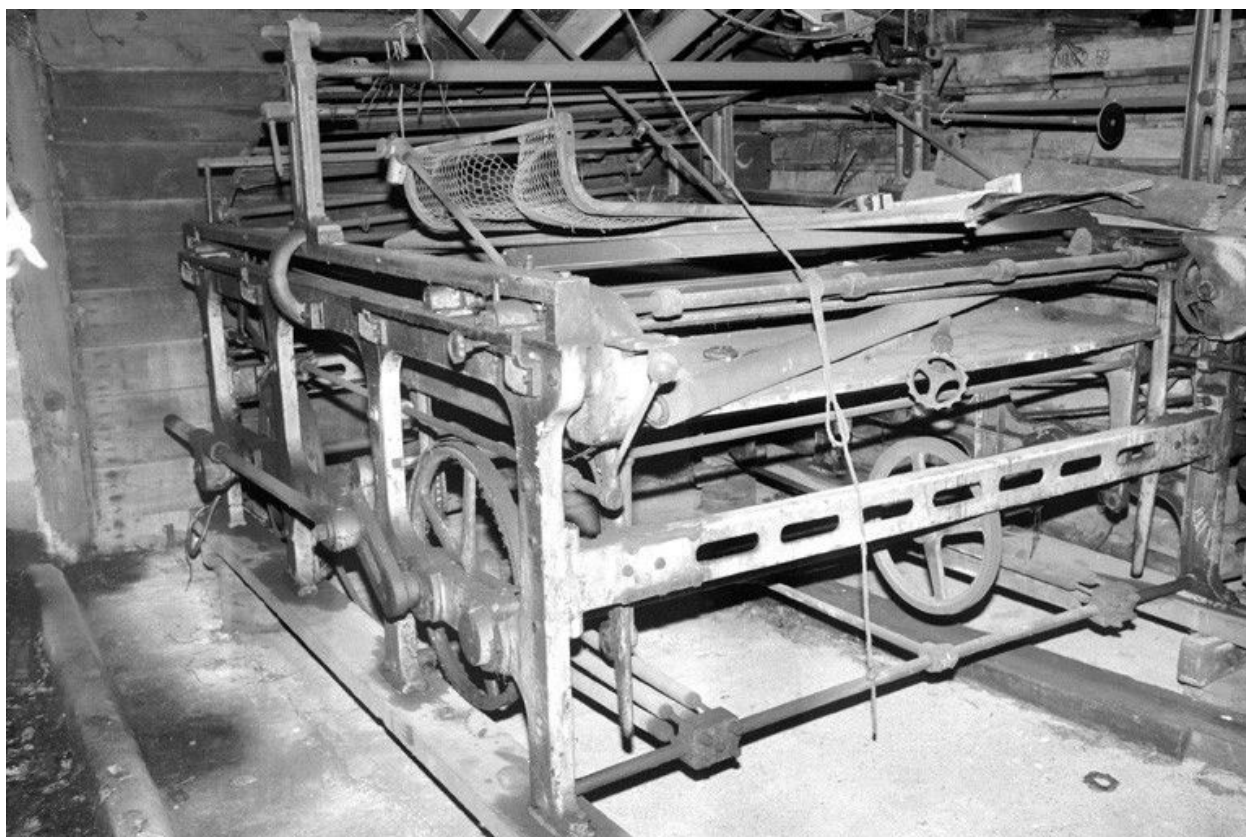
Plieuse. La plaque porte la mention : (IRION-VOSSELER) Scweningen et Rogo (Mulhouse), sans date
