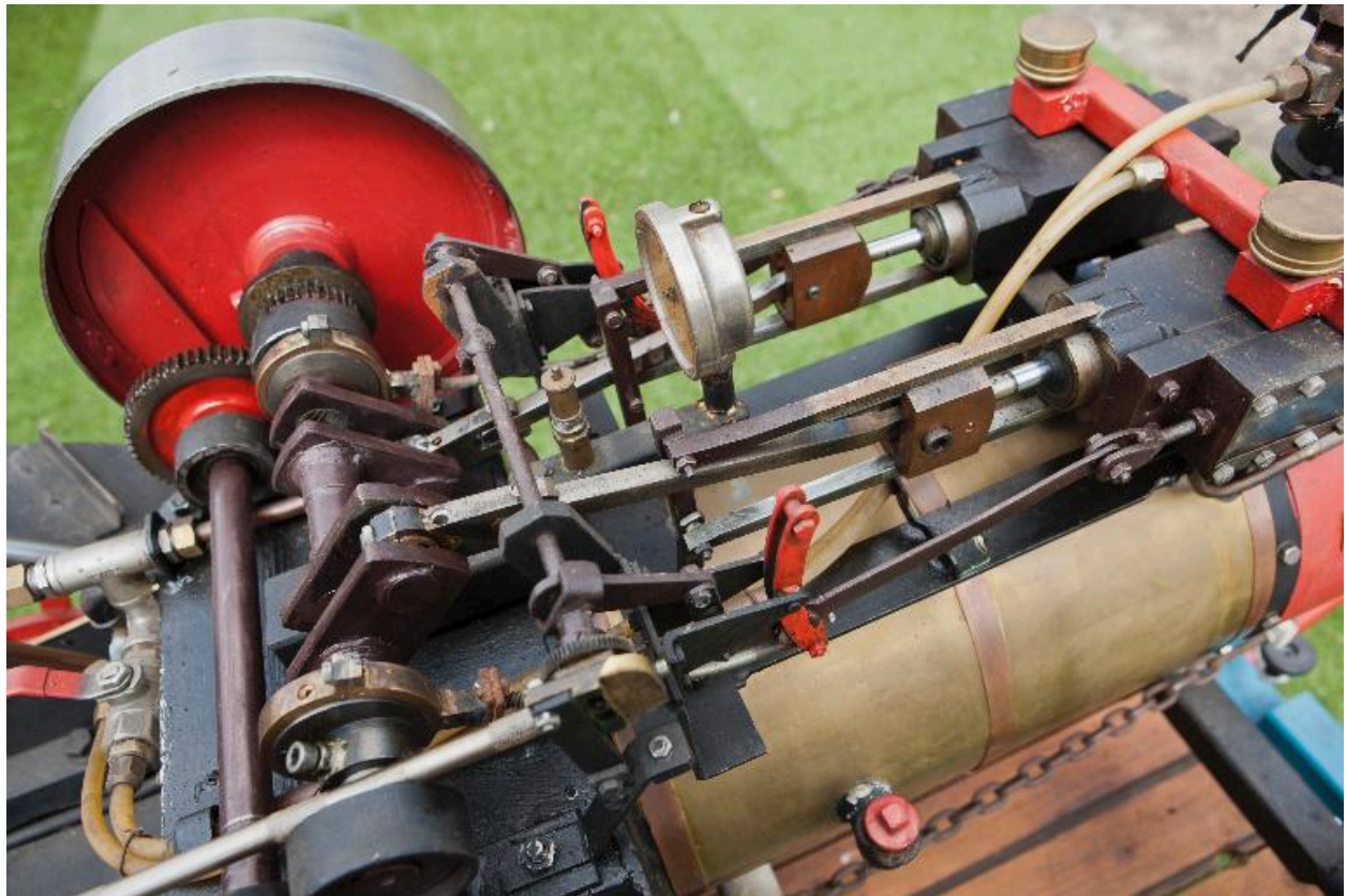
Locomobile, détail.
