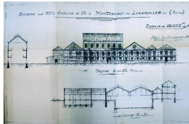
Coupes et élévation de la sucrerie Séblin, 1er juillet 1918. (AD Aisne ; 15 R 1819/2).
