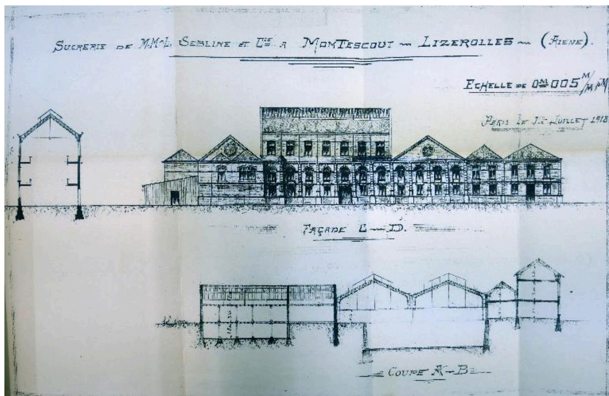
Coupes et élévation de la sucrerie Séblin, 1er juillet 1918. (AD Aisne ;15 R 1819/2).
