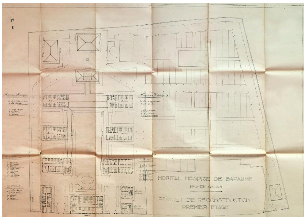
Hôpital - hospice de Bapaume - Pas-de-Calais : projet de reconstruction. Feuille 12 C : 1er étage. Ni signé ni daté. (AD Pas-de-Calais, X1174).
