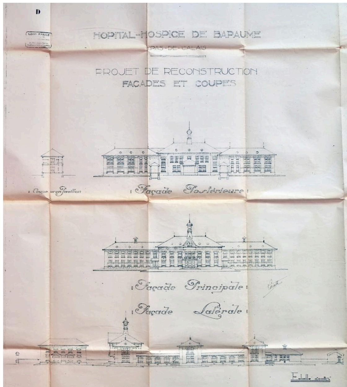
Hôpital - hospice de Bapaume - Pas-de-Calais : projet de reconstruction. Feuille 12 D : façades et coupes : façade postérieure ; façade principale ; façade latérale ; coupe sur un pavillon. Timbre et signature de l'architecte Louis Faille. Sans date. (AD Pas-de-Calais, X1174).
