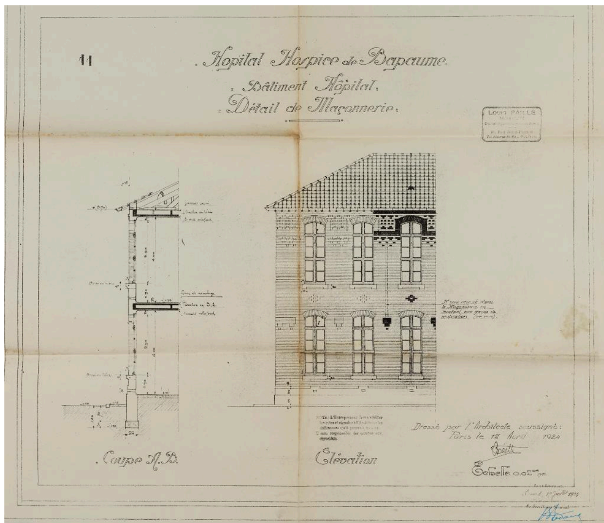
Hôpital - hospice de Bapaume. Projet de reconstruction : bâtiment hôpital : détail de la maçonnerie : coupe AB, élévation. Daté et signé par Louis Faille, architecte, le 1er avril 1924. Validé par le secrétaire général le 10 juillet 1924. (AD Pas-de-Calais, X1175).
