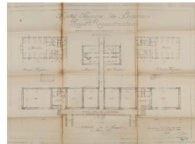
Hôpital - hospice de Bapaume. Projet de reconstruction : bâtiment de l'hospice : plans du sous-sol et de l'étage ; plan du sous-sol de la cuisine. Daté et signé par Louis Faille, architecte, le 1er avril 1924. Validé par le secrétaire général le 10 juillet 1924. (AD Pas-de-Calais, X1175). Phot. Thibaut Pierre (reproduction) IVR32_20216200172NUCA
