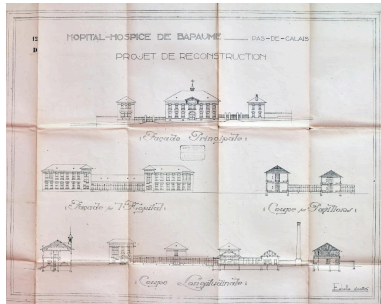
Hôpital - hospice de Bapaume - Pas-de-Calais : projet de reconstruction. Feuille 12 D : façade principale ; façade sur l'hôpital ; coupe sur pavillons ; coupe longitudinale. Ni signé ni daté. (AD Pas-de-Calais, X1174). Phot. Thibaut Pierre (reproduction) IVR32_20216200002NUCA
