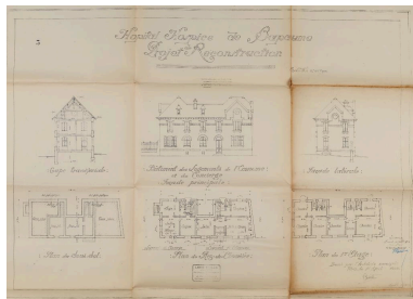
Hôpital - hospice de Bapaume. Projet de reconstruction : bâtiment des logements de l'économe et du concierge : coupe transversale ; façade principale ; façade latérale ; plans du sous-sol, du rez-de-chaussée et de l'étage. Daté et signé par Louis Faille, architecte, le 1er avril 1924. Validé par le secrétaire général le 10 juillet 1924. (AD Pas-de-Calais, X1175). Phot. Thibaut Pierre (reproduction) IVR32_20216200169NUCA
