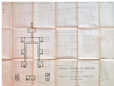
Hôpital - hospice de Bapaume - Pas-de-Calais : projet de reconstruction. Feuille 12 A : sous-sol. Timbre de l'architecte Louis Faille. Ni signé ni daté. (AD Pas-de-Calais, X1174). Phot. Thibaut Pierre (reproduction) IVR32_20216200005NUCA
