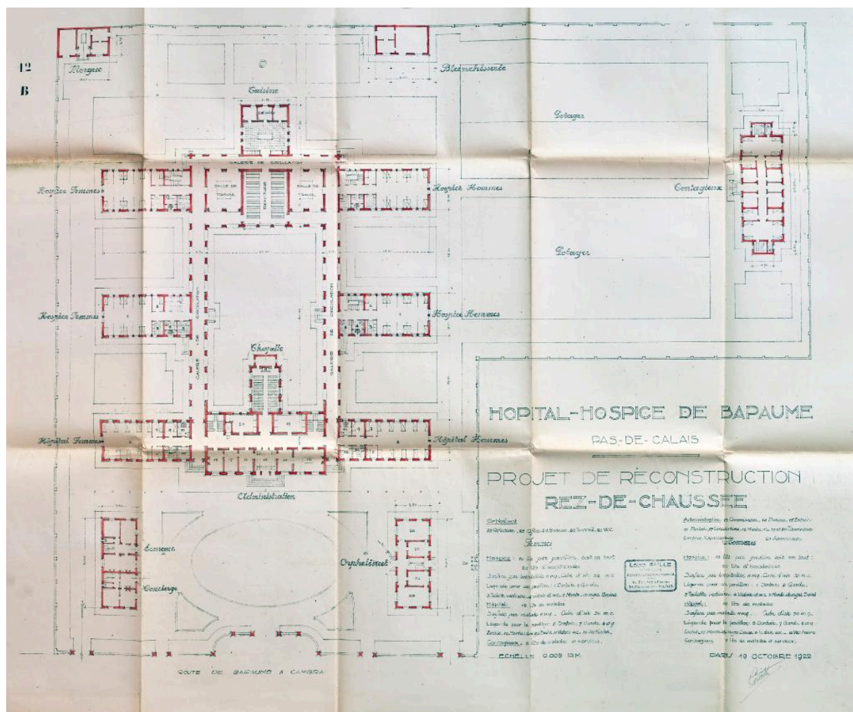
Hôpital - hospice de Bapaume - Pas-de-Calais : projet de reconstruction. Feuille 12 B : rez-de-chaussée. Timbre et signature de l'architecte Louis Faille. Daté du 19 octobre 1922. (AD Pas-de-Calais, X1174).
