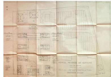
Hôpital - hospice de Bapaume - Pas-de-Calais : projet de reconstruction. Feuille 12 C : 1er étage. Ni signé ni daté. (AD Pas-de-Calais, X1174). Phot. Thibaut Pierre (reproduction) IVR32_20216200006NUCA
