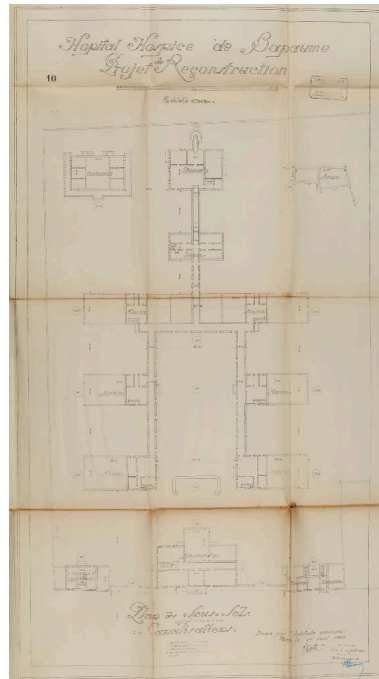
Hôpital - hospice de Bapaume. Projet de reconstruction : plan des sous-sols et canalisations. Daté et signé par Louis Faille, architecte, le 1er avril 1924. Validé par le secrétaire général le 10 juillet 1924. (AD Pas-de-Calais, X1175). Phot. Thibaut Pierre (reproduction) IVR32_20216200177NUCA
