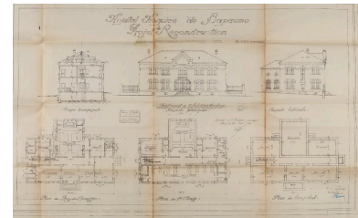
Hôpital - hospice de Bapaume. Projet de reconstruction : bâtiment de l'administration : coupe transversale ; façade principale ; façade latérale ; plans du sous-sol, du rez-de-chaussée et de l'étage. Daté et signé par Louis Faille, architecte, le 1er avril 1924. Validé par le secrétaire général le 10 juillet 1924. (AD Pas-de-Calais, X1175). Phot. Thibaut Pierre (reproduction) IVR32_20216200171NUCA
