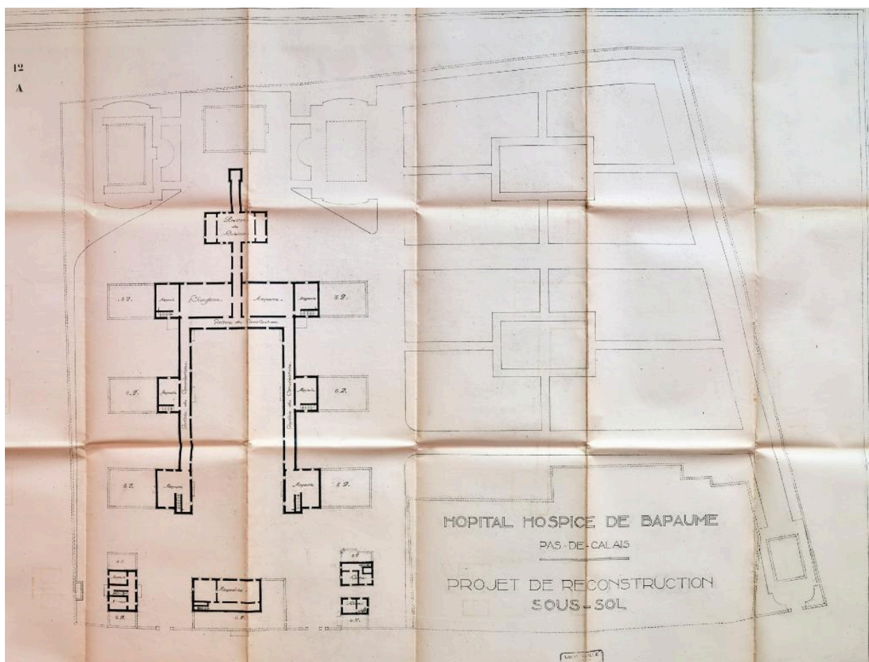
Hôpital - hospice de Bapaume - Pas-de-Calais : projet de reconstruction. Feuille 12 A : sous-sol. Timbre de l'architecte Louis Faille. Ni signé ni daté. (AD Pas-de-Calais, X1174).
