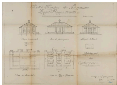
Hôpital - hospice de Bapaume. Projet de reconstruction : bâtiment des contagieux : coupe transversale ; façade principale ; façade latérale ; plans du sous-sol et du rez-de-chaussée. Daté et signé par Louis Faille, architecte, le 1er avril 1924. Validé par le secrétaire général le 10 juillet 1924. (AD Pas-de-Calais, X1175). Phot. Thibaut Pierre (reproduction) IVR32_20216200170NUCA
