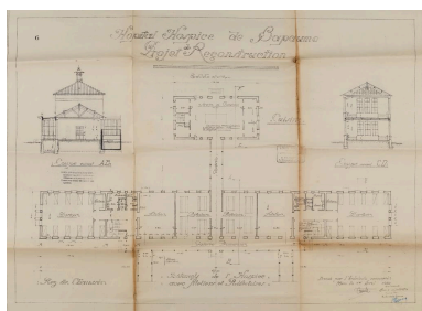
Hôpital - hospice de Bapaume. Projet de reconstruction : bâtiment de l'hospice avec ateliers et réfectoire : coupe suivant AB ; coupe suivant CD ; plans du rez-de-chaussée.
