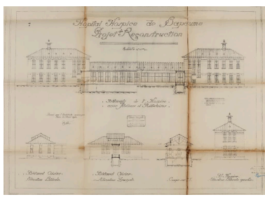
Hôpital - hospice de Bapaume. Projet de reconstruction : bâtiment de l'hospice avec ateliers et réfectoire : façade principale ; bâtiment cuisine : façade latérale, élévation principale, coupe sur EF ; bâtiment hospice : élévation latérale gauche. Daté et signé par Louis Faille, architecte, le 1er avril 1924. Validé par le secrétaire général le 10 juillet 1924. (AD Pas-de-Calais, X1175).
