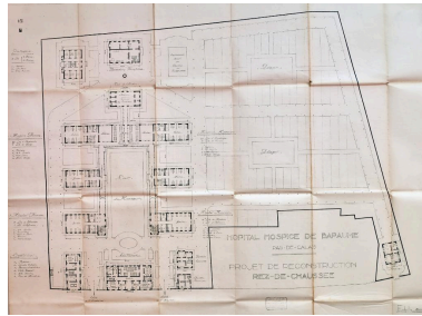
Hôpital - hospice de Bapaume - Pas-de-Calais : projet de reconstruction. Feuille 12 B : rez-de-chaussée. Timbre de l'architecte Louis Faille. Ni signé ni daté. (AD Pas-de-Calais, X1174). Phot. Thibaut Pierre (reproduction) IVR32_20216200004NUCA
