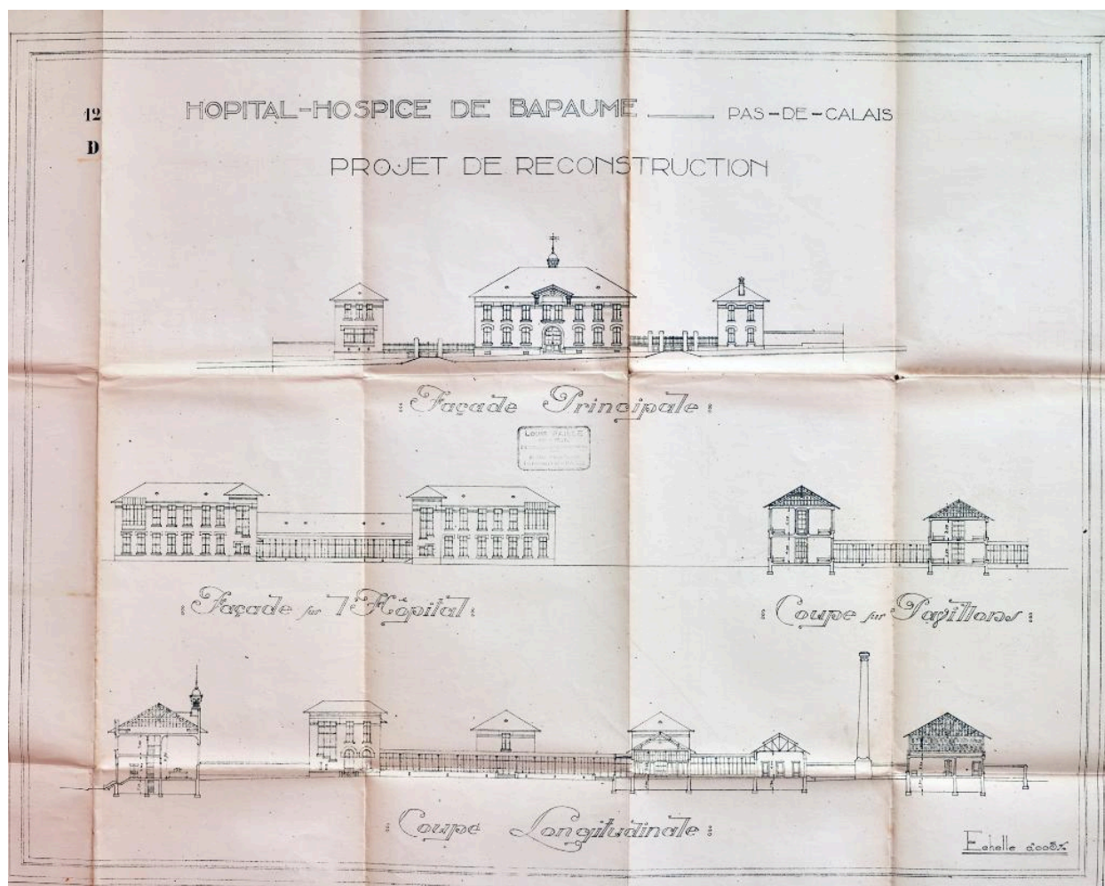
Hôpital - hospice de Bapaume - Pas-de-Calais : projet de reconstruction. Feuille 12 D : façade principale ; façade sur l'hôpital ; coupe sur pavillons ; coupe longitudinale. Ni signé ni daté. (AD Pas-de-Calais, X1174).
