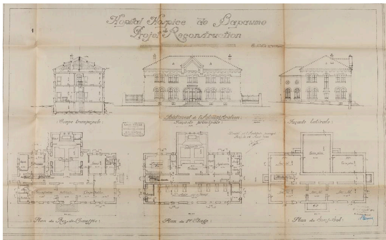
Hôpital - hospice de Bapaume. Projet de reconstruction : bâtiment de l'administration : coupe transversale ; façade principale ; façade latérale ; plans du sous-sol, du rez-de-chaussée et de l'étage. Daté et signé par Louis Faille, architecte, le 1er avril 1924. Validé par le secrétaire général le 10 juillet 1924. (AD Pas-de-Calais, X1175).
