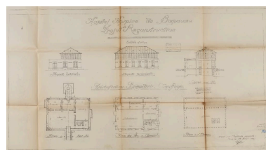
Hôpital - hospice de Bapaume. Projet de reconstruction : bâtiment de la désinfection - buanderie - chauffage : façade latérale ; façade principale ; coupe sur GH ; plans du sous-sol, du rez-de-chaussée et de l'étage. Daté et signé par Louis Faille, architecte, le 1er avril 1924. Validé par le secrétaire général le 10 juillet 1924. (AD Pas-de-Calais, X1175). Phot. Thibaut Pierre (reproduction) IVR32_20216200167NUCA
