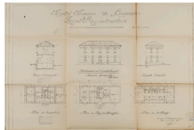
Hôpital - hospice de Bapaume. Projet de reconstruction : bâtiment de l'orphelinat : coupe transversale ; façade principale ; façade latérale ; plans du sous-sol, du rez-de-chaussée et de l'étage. Daté et signé par Louis Faille, architecte, le 1er avril 1924. Validé par le secrétaire général le 10 juillet 1924. (AD Pas-de-Calais, X1175). Phot. Thibaut Pierre (reproduction) IVR32_20216200174NUCA
