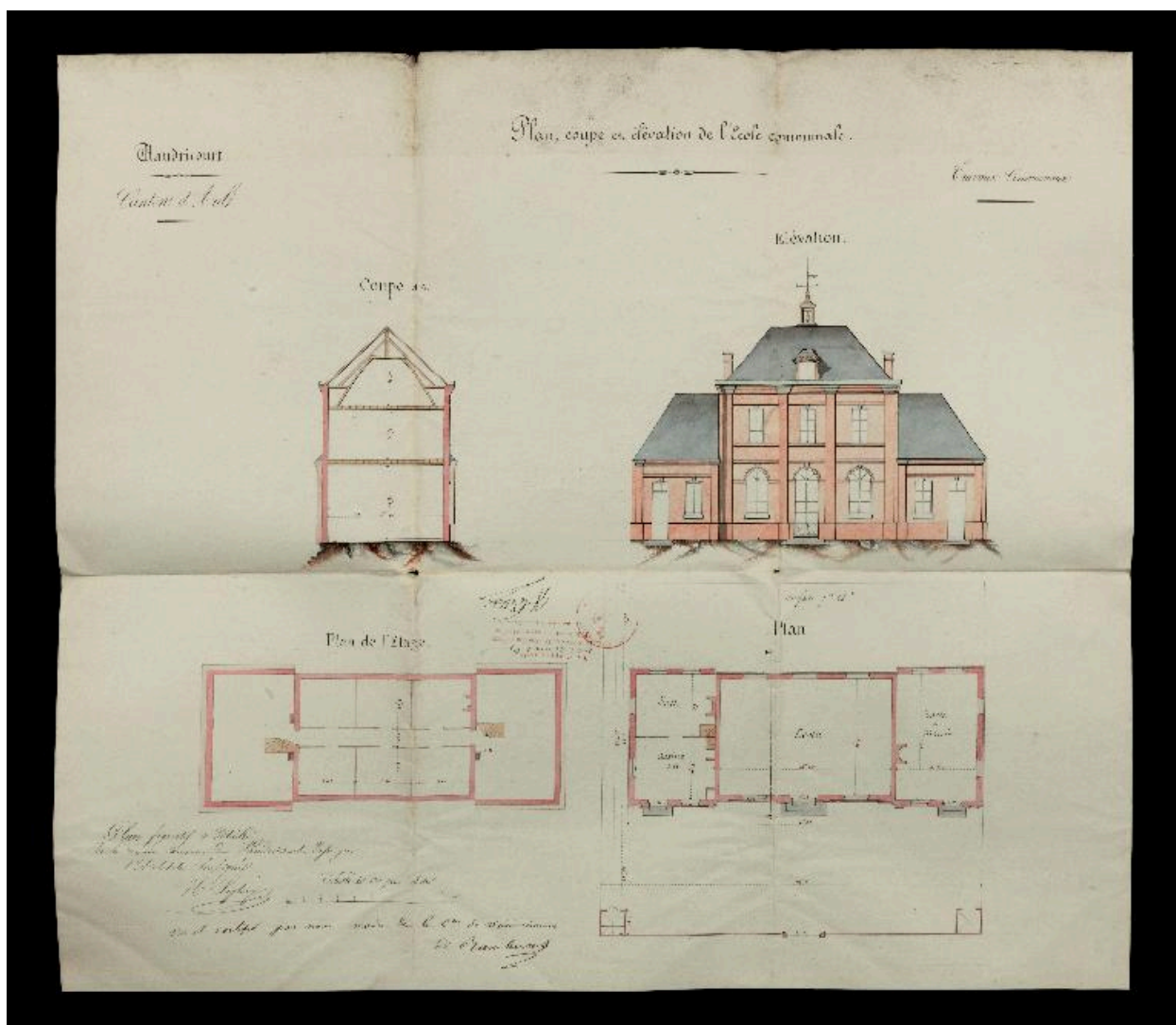
Plan, coupe et élévation de l'école et mairie, Lephy architecte, 1862 (AD Somme ; 99 O 3660).
