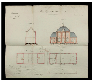
Plan, coupe et élévation de l'école et mairie, Lephay architecte, 1862 (AD Somme ; 99 O 3660). Phot. Thierry Lefébure IVR22_20128001246NUC2A
