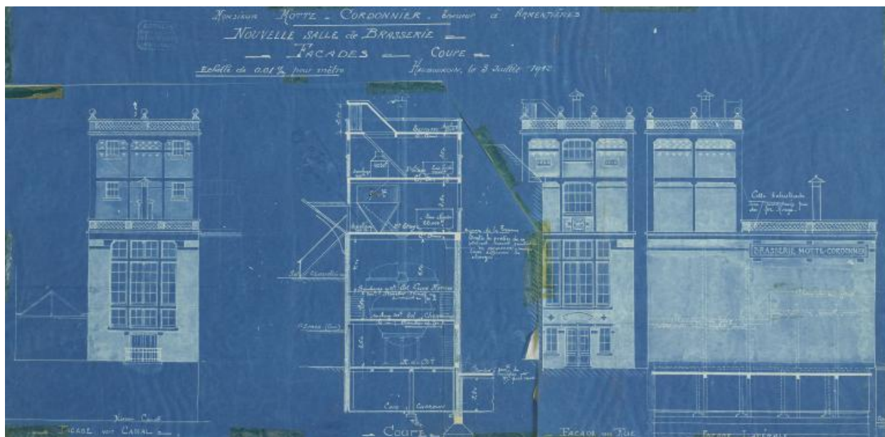
Nouvelle salle de brasserie de M. Motte-Cordonnier, brasseur à Armentières. Coupe et élévations, Gustave Defretin architecte, 3 juillet 1912 (AP Motte-Cordonnier).
