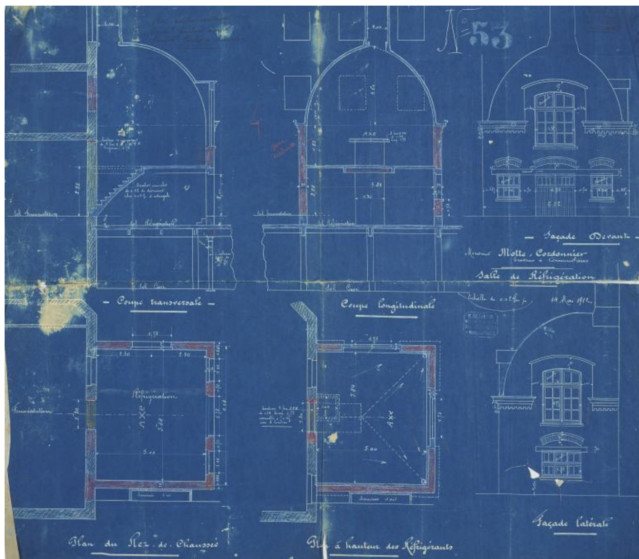
Salle des réfrigérants de la brasserie de M. Motte-Cordonnier, brasseur à Armentières. Coupes, Gustave Defretin architecte, 14 mai 1912 (AP Motte-Cordonnier).
