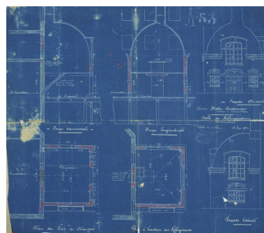
Salle des réfrigérants de la brasserie de M. Motte-Cordonnier, brasseur à Armentières. Coupes, Gustave Defretin architecte, 14 mai 1912 (AP Motte-Cordonnier). Repro. Delphine Volto-Jourdan IVR32_20215900010NUCA
