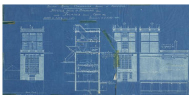
Nouvelle salle de brasserie de M. Motte-Cordonnier, brasseur à Armentières. Coupe et élévations, Gustave Defretin architecte, 3 juillet 1912 (AP Motte-Cordonnier). Repro. Delphine Volto-Jourdan IVR32_20215900011NUCA
