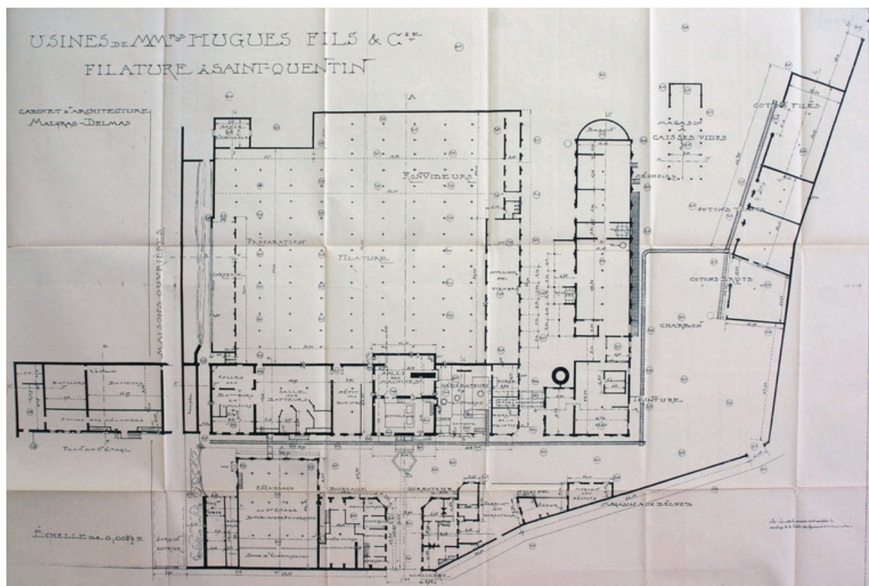
Plan des ateliers en 1914, par Malgras-Delmas (AD Aisne).
