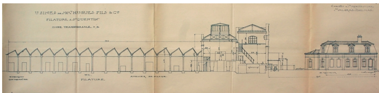
Coupe transversale de la filature en 1914, par Malgras-Delmas (AD Aisne).
