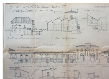
Façades et coupes de la filature en 1914, par Malgras-Delmas (AD Aisne).
