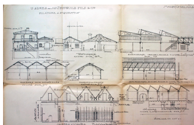
Façades et coupes de la filature en 1914, par Malgras-Delmas (AD Aisne).
