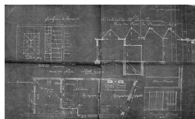
Plans, coupes, élévations de la teinturerie projetée par M. Detollenaere, 1920 (AD Nord ; M 41710401). Repro. Philippe Dapvril IVR31_19875902154XB
