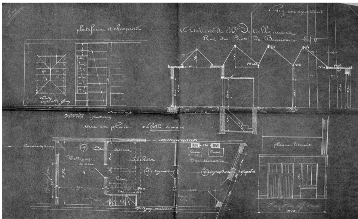
Plans, coupes, élévations de la teinturerie projetée par M. Detollenaere, 1920 (AD Nord ; M 41710401).
