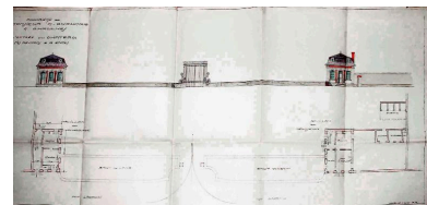
L'entrée du château, les pavillons et la grille : plan et élévation, A. Lefèvre (AD Somme ; 10 R 307). Phot. Gilles-Henri Bailly (reproduction) IVR22_20158005215NUCA
