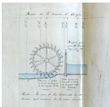
La roue hydraulique de la scierie en 1823 (AD Oise ; 9Sp182).
