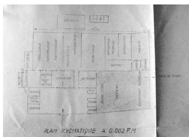
Plan de la société des Tricotages de l'Oise et des agrandissements projetés, 1948 (AC Montataire ; 102W1). Phot. Clarisse Lorieux (reproduction) IVR22_20086005088NUCAB
