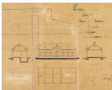
Projet pour la construction d'une école mixte, mairie, logement d'instituteur, par Léopold Digeon, 15 décembre 1868 (AD Somme ; 99 O 1507). Repro. Thierry Lefébure
