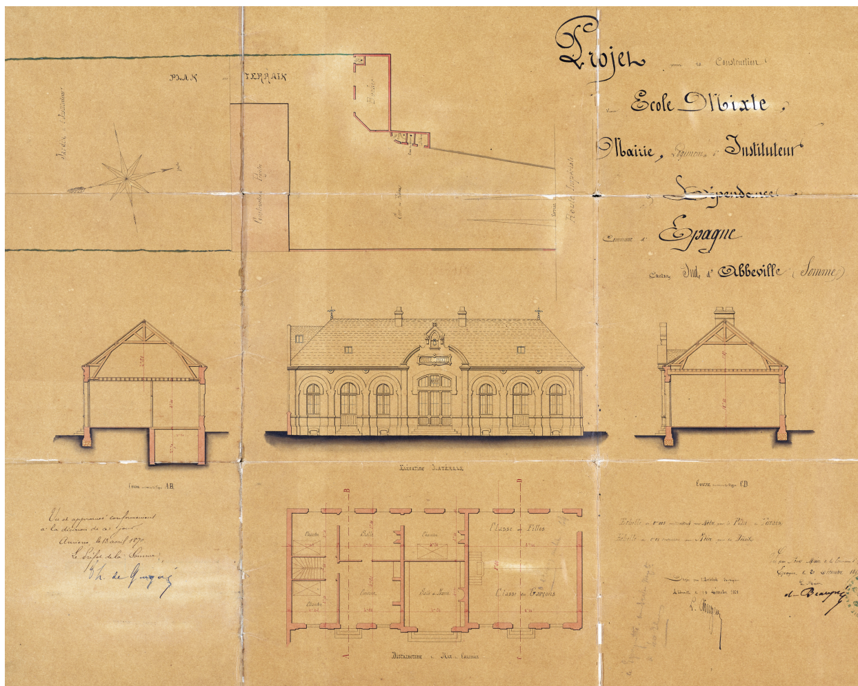
Projet pour la construction d'une école mixte, mairie, logement d'instituteur, par Léopold Digeon, 15 décembre 1868 (AD Somme ; 99 O 1507).
