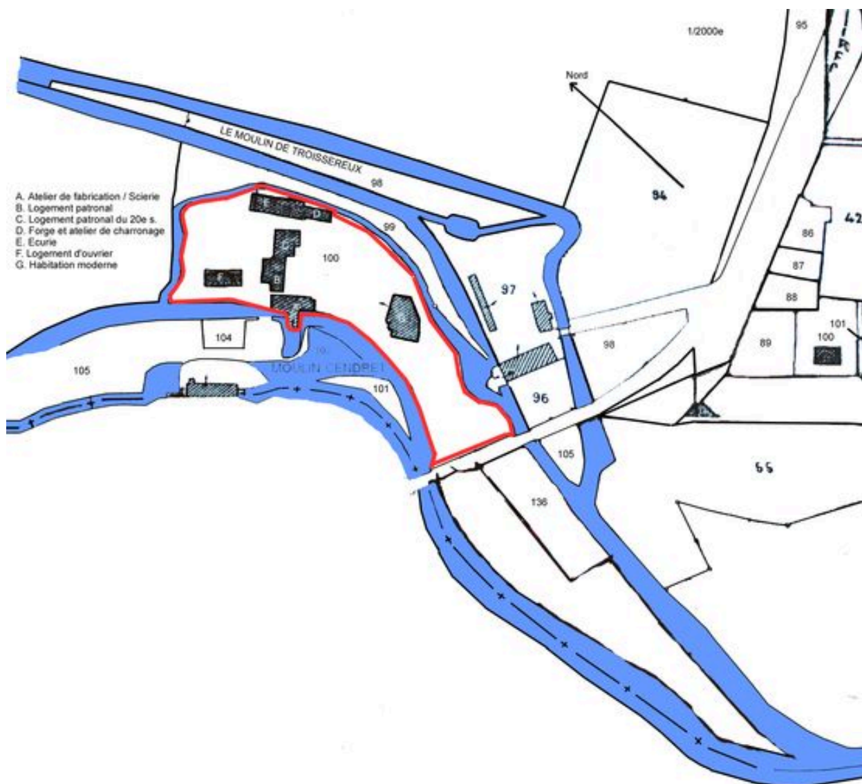
Plan cadastral de la scierie, section ZL, avec indication des différentes fonctions de bâtiments.
