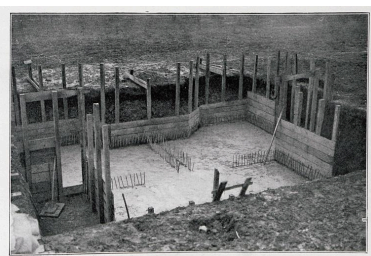
Le coffrage extérieur est achevé et la semelle coulée. In: Deutsche Frontbauarbeit im Kriege, p.129 Phot. Staatsbibliothek zu Berlin (reproduction) IVR32_20176200527NUCA
