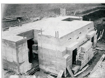
L'édifice débarrassé de son coffrage. in: Deutsche Frontbauarbeit im Kriege, p.137 Phot. Staatsbibliothek zu Berlin (reproduction) IVR32_20176200535NUCA
