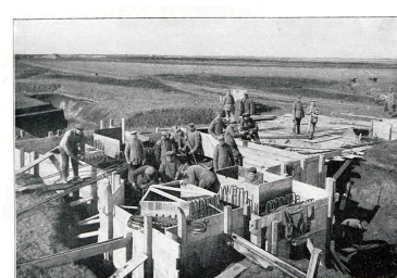
Coffrage des murs de l'édifice. In: Deutsche Frontbauarbeit im Kriege, p.130 Phot. Staatsbibliothek zu Berlin (reproduction) IVR32_20176200529NUCA
