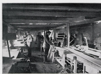
Atelier de menuiserie. Ici sont façonnés les éléments de coffrage. in: Deutsche Frontbauarbeit im Kriege, p.128 Phot. Staatsbibliothek zu Berlin (reproduction) IVR32_20176200524NUCA
