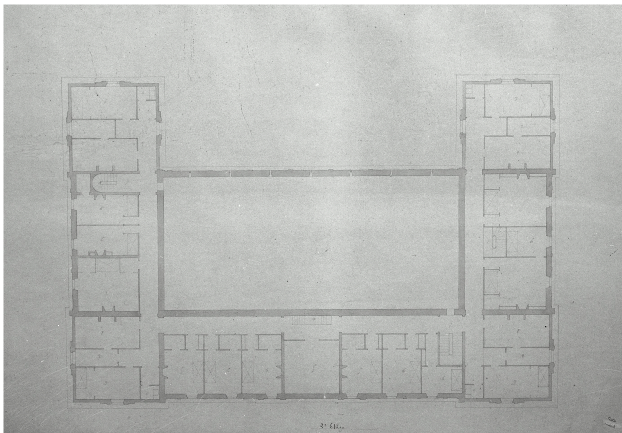
Etablissement de bains, casino, projet 1861, pl. 87, plan du 2e étage. B.M. Boulogne-sur-Mer, mss. 535 P.
