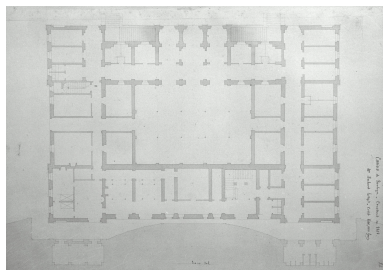
Etablissement de bains, casino, projet 1861, pl. 84, plan du sous-sol. B.M. Boulogne-sur-Mer, mss. 535 P. Repro. Caudroit Philippe IVR31_19846200198X
