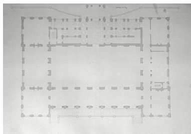
Etablissement de bains, casino, projet 1861, pl. 85, plan du rez-de-chaussée. B.M. Boulogne-sur-Mer, mss. 535 P. Repro. Caudroit Philippe IVR31_19846200196X
