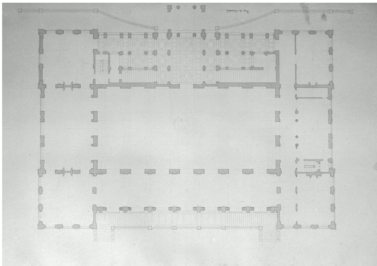
Etablissement de bains, casino, projet 1861, pl. 85, plan du rez-de-chaussée. B.M. Boulogne-sur-Mer, mss. 535 P.
