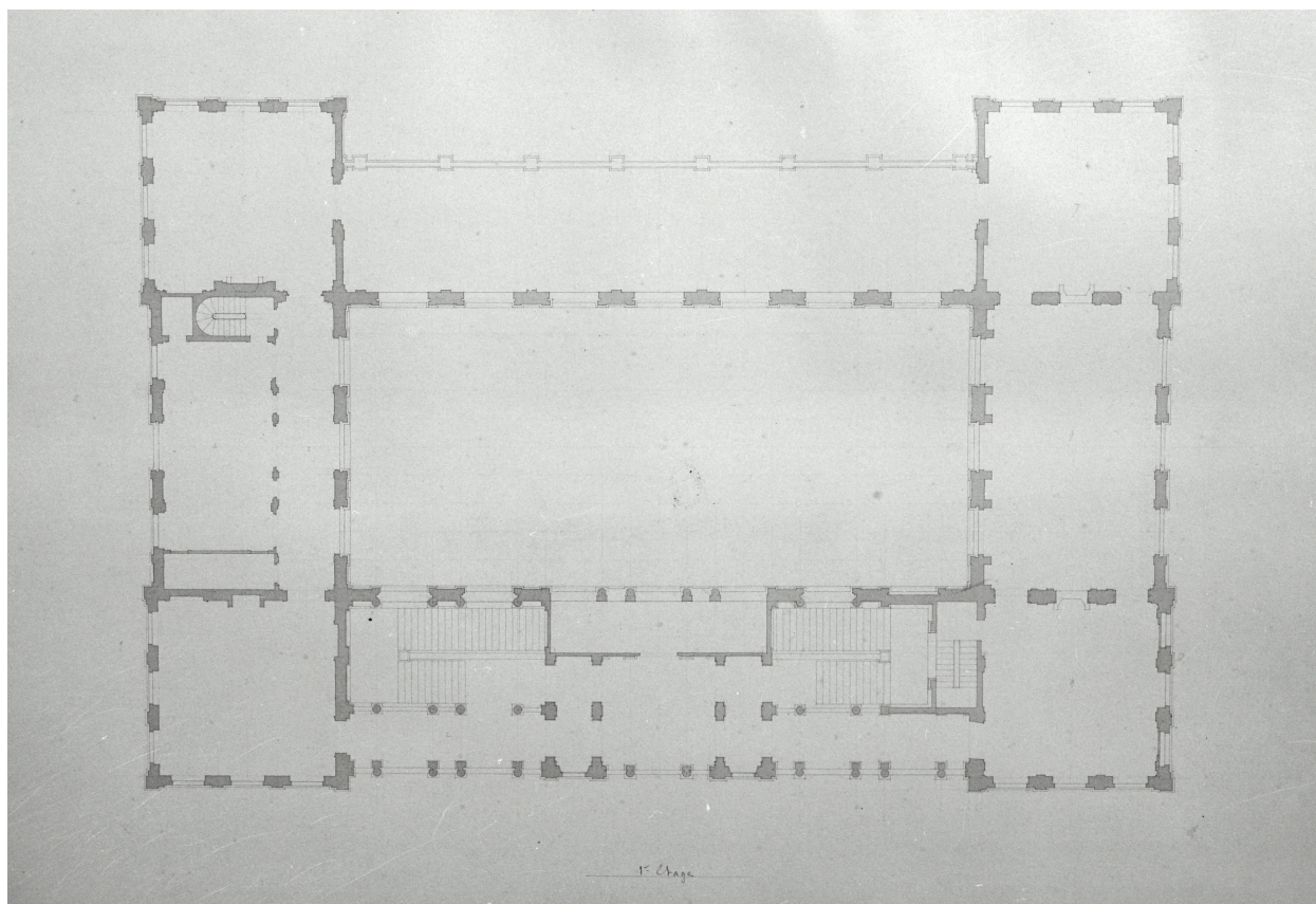
Etablissement de bains, casino, projet 1861, pl. 86, plan du 1er étage. B.M. Boulogne-sur-Mer, mss. 535 P.
