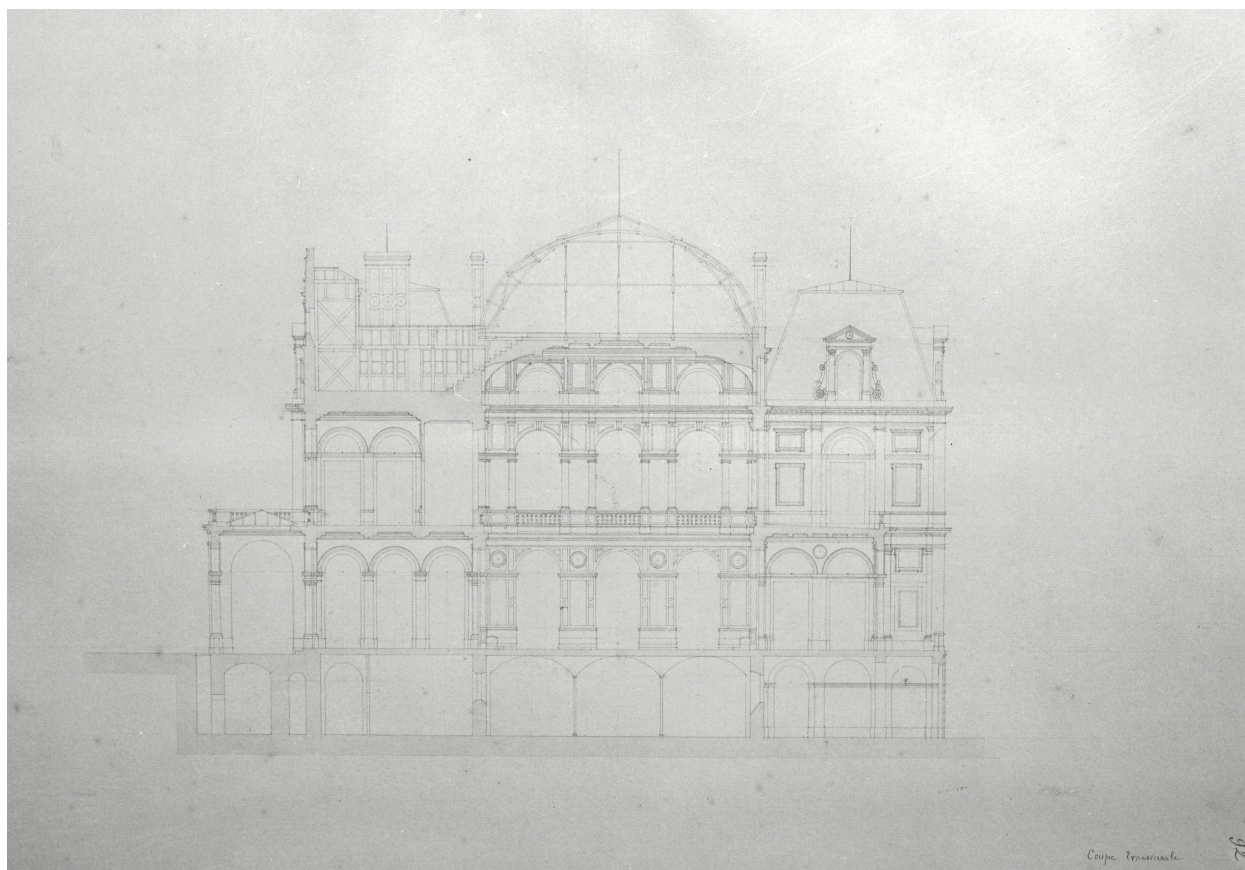
Etablissement de bains, casino, projet 1861, pl. 92, coupe transversale. B.M. Boulogne-sur-Mer, mss. 535 P.
