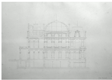
Etablissement de bains, casino, projet 1861, pl. 92, coupe transversale. B.M. Boulogne-sur-Mer, mss. 535 P. Repro. Caudroit Philippe IVR31_19846200189X
