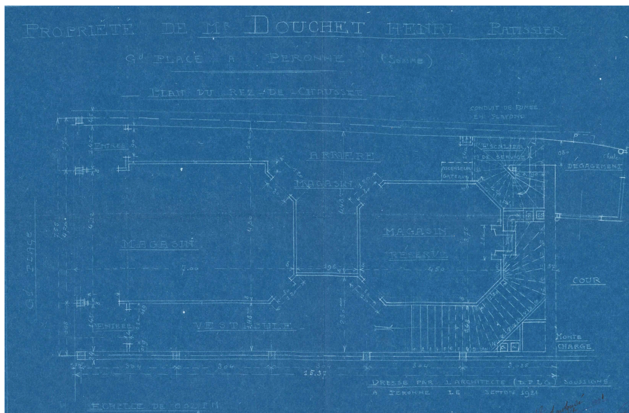
Propriété de M. Douchet Henri. Pâtissier. Grand Place à Péronne. Plan du rez-de-chaussée, Daniel Roguet architecte, 1921 (AD Somme ; 10R 1022).
