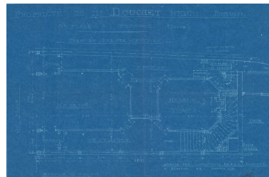
Propriété de M. Douchet Henri. Pâtissier. Grand Place à Péronne. Plan du rez-de- chaussée, Daniel Roguet architecte, 1921 (AD Somme ; 10R 1022). Phot. Archives départementales de la Somme IVR32_20228005147NUCA
