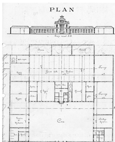
Plan et élévation d'une imprimerie (AD Oise ; fonds Silvert, 471-1895). Phot. Monnehay-Vulliet Marie-Laure IVR22_20096000533NUCA
