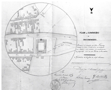
Plan de commando et incommodo annexé à la demande du sieur Lescornez tendant à obtenir l'autorisation de construire une brasserie avec machine et générateur..., 1879 (AC Armentières ; 1.777.51). Repro. Olivier Marlard IVR31_19885901289X
