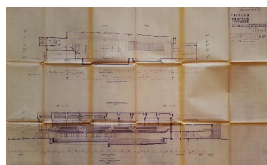
Avant-projet de piscine olympique couverte : coupes transversale et longitudinale, André Evard architecte, 1967-1968 (AN ; 19800382/234). Repro. Laurence Schlosser IVR32_20176205038NUCA
