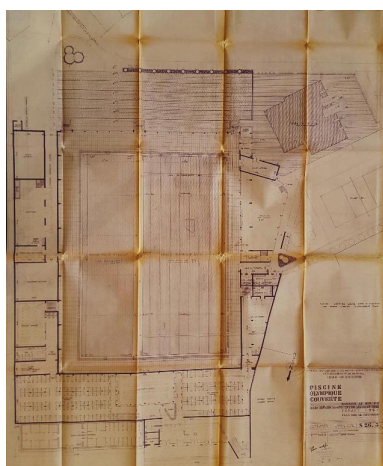
Avant-projet de piscine olympique couverte : plan de rez-de-chaussée, André Evard architecte, 1967-1968 (AN ; 19800382/234). Repro. Laurence Schlosser IVR32_20176205036NUCA
