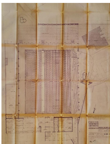
Avant-projet de piscine olympique couverte : plan d'étage, André Evard architecte, 1967-1968 (AN ; 19800382/234). Repro. Laurence Schlosser IVR32_20176205037NUCA
