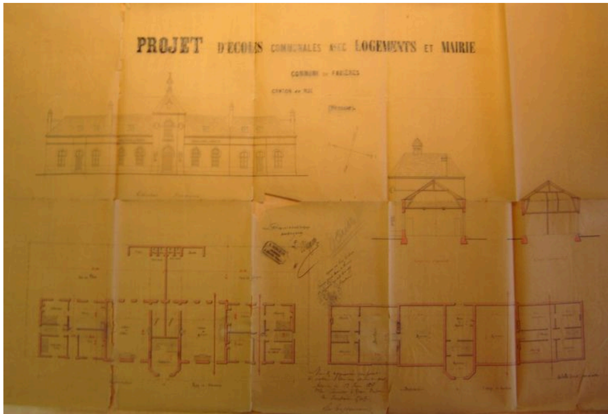
Plan, coupe et élévation du projet de 1865.
