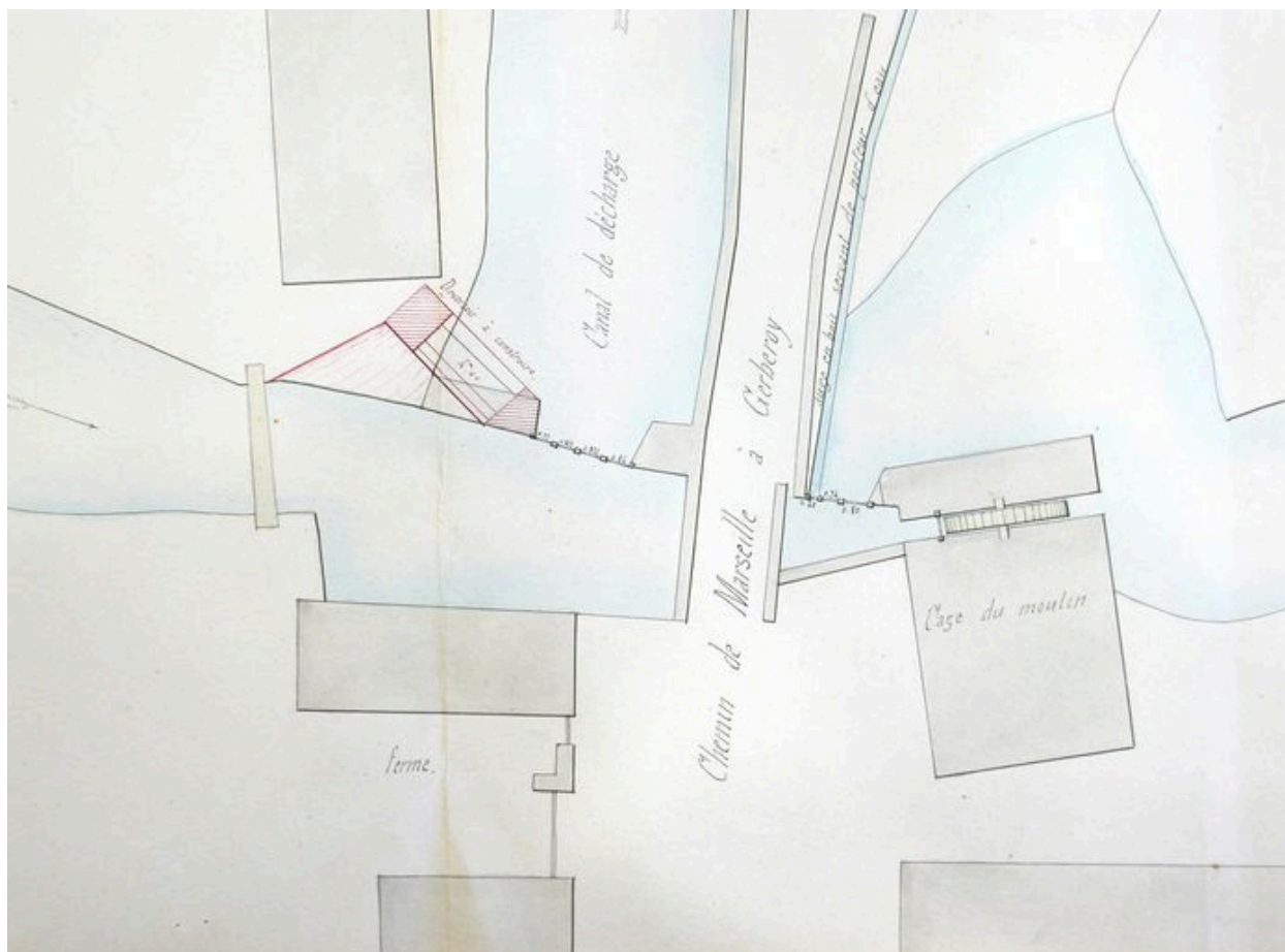
Plan détaillé du moulin de Lachapelle, appartenant à M. de Songeon, 3 août 1852.
