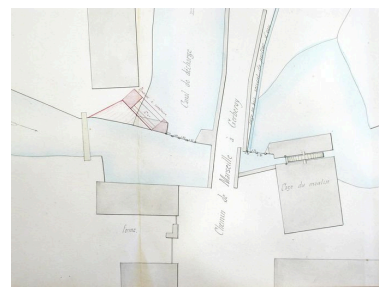
Plan détaillé du moulin de Lachapelle, appartenant à M. de Songeons, 3 août 1852. Phot. Fournier Bertrand (reproduction)
