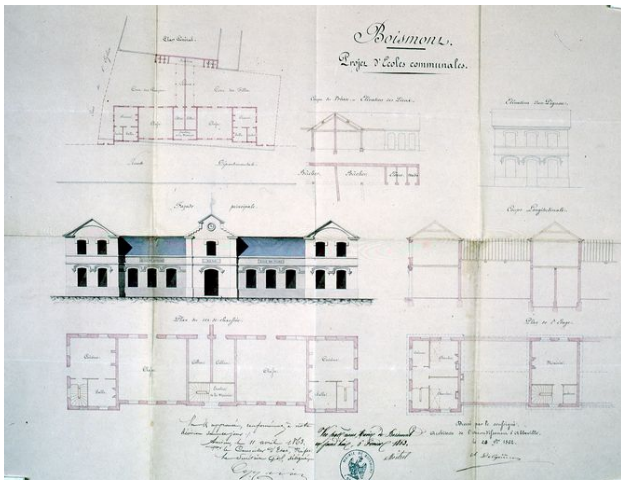
Plan, coupe et élévation du projet de construction d'une mairie école à Boismont, Charles Delignières, 1862.
