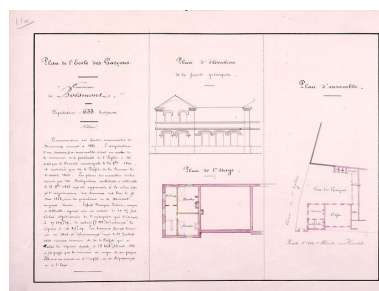
Plan définitif de l'école des garçons, par Charles Delignières. Phot. Monnehay-Vulliet Marie-Laure
