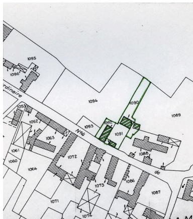
Plan de situation. Extrait du plan cadastral de 1962, section B4 1090, 1091, 1092.. Repro. Monnehay-Vulliet Marie- Laure , Autr. Michel Hérold IVR22_20096000098NUCA
