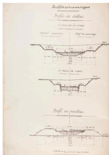
Profils en travers type, profil en déblai, profil en remblai. Notice sur l'avant-projet par G. La Rivière et D. Bourgeois, bassin houiller du Nord et du Pas-du-Calais, Exposition internationale universelle de Liège 1905, Lille, imprimerie Danel, 1905 (AD Pas-de-Calais ; S651 : 3S3326). Repro. Hubert Bouvet IVR32_20186200077NUC4A
