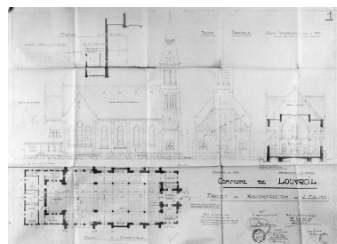
Élévation latérale, antérieure et coupe transversale par Paul Vilain (1860-1933), architecte, 9 août 1929 (AD Nord ; O 371/148). Phot. Thierry Petitberghien IVR31_20015901975V
