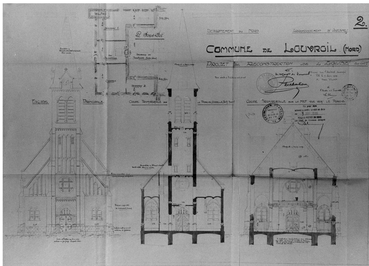
Élévation antérieure et coupes par Paul Vilain (1860-1933), architecte, aout 1929 (AD Nord ; O371/148).
