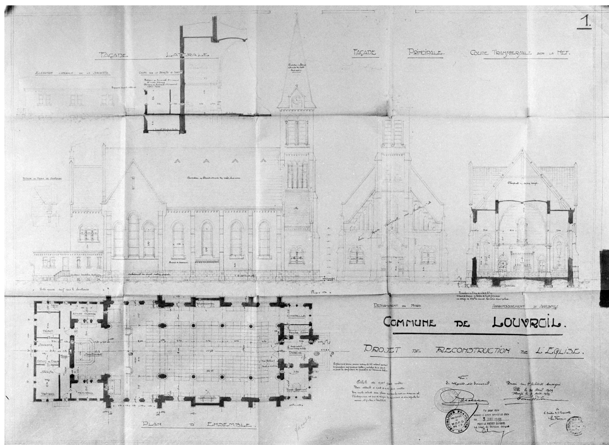
Élévation latérale, antérieure et coupe transversale par Paul Vilain (1860-1933), architecte, 9 août 1929 (AD Nord ; O 371/148).
