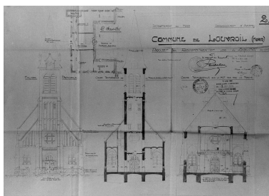
Élévation antérieure et coupes par Paul Vilain (1860-1933), architecte, 9 août 1929 (AD Nord ; O371/148). Phot. Thierry Petitberghien IVR31_20015901912X
