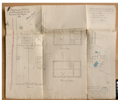
Chepoix (Oise). Plan du projet d'école mixte avec logement de l'instituteur, 1864 (AD Oise).
