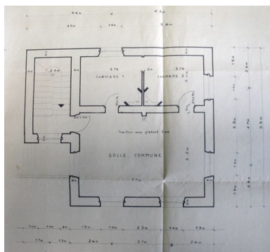
Plan de masse du pavillon du château transformé en chambres d'ouvriers en 1958 (AC Villers-Saint-Paul ; 44W20). Phot. Clarisse Lorieux (reproduction) IVR22_20096005139NUCAB
