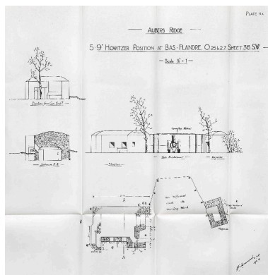
Plans et coupe d'une des deux positions d'artillerie (casemate est, n° 135, IA59004842) in : Studies of German defences near Lille : Pl. 6a du 31/01/1919 Phot. Pierre Thibaut (reproduction) IVR32_20165901722NUCA
