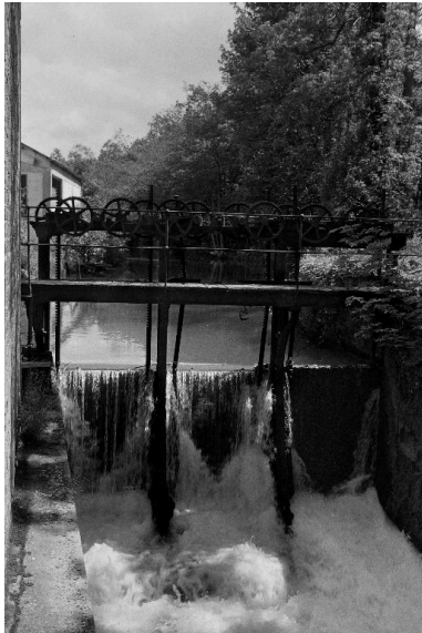
Vannes de décharge. Phot. Benoît Dufournier IVR22_19878000012Z
