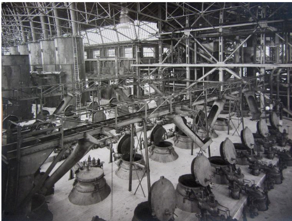
Les vases de diffusion de la sucrerie, 6 novembre 1922 (AD Somme ; 49 Fi 18).
