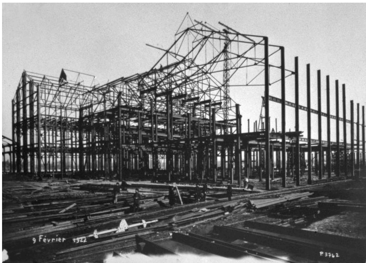
Structure métallique du grand atelier de fabrication de la sucrerie, 9 février 1922 (Archives privées de l'entreprise).
