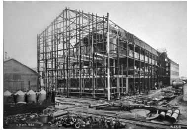
Structure métallique du grand atelier de fabrication, 2 août 1922 (Archives privées de l'entreprise). Phot. Bertrand Fournier IVR22_20008000405ZA
