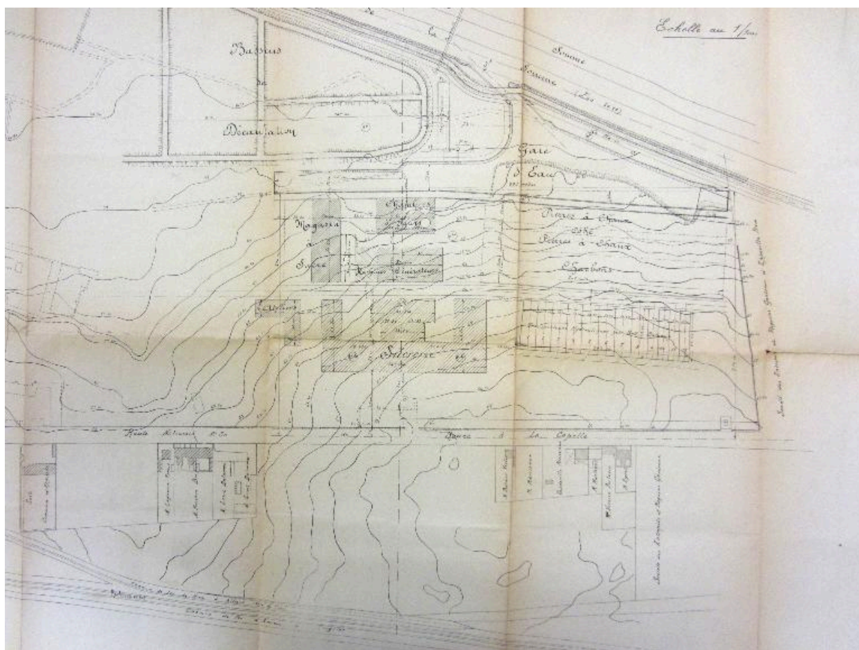
Plan d'ensemble de la sucrerie centrale d'Eppeville, avec indications des courbes de niveau, 1921. (AD Somme ; 5 M 624).
