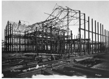
Structure métallique du grand atelier de fabrication de la sucrerie, 9 février 1922 (Archives privées de l'entreprise). Phot. Bertrand Fournier IVR22_20008000404ZA
