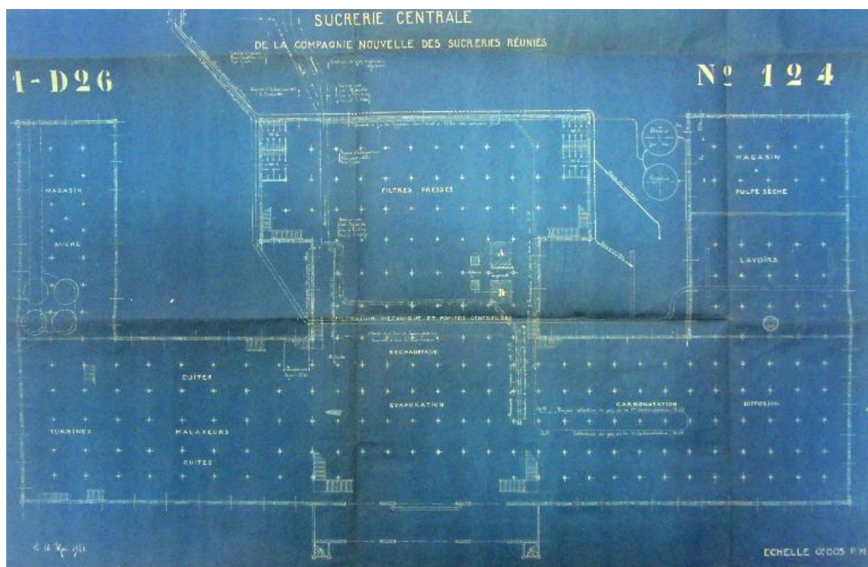
Plan détaillé de l'atelier principal de la sucrerie, 19 mai 1921 (AD Somme ; 5 M 623).
