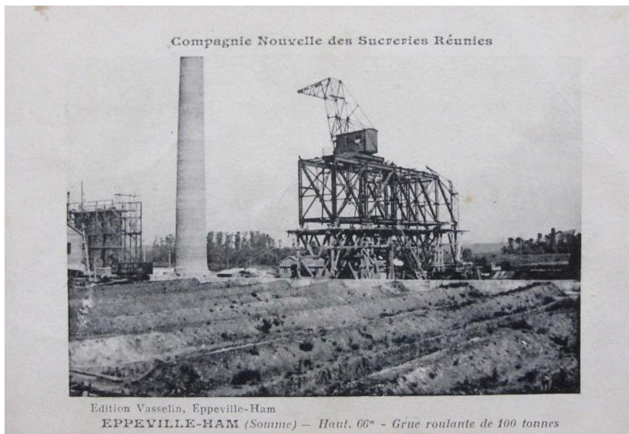
La grue roulante de 100 tonnes. Carte postale, 1922 (Coll. Cercle Cartophile de Ham).
