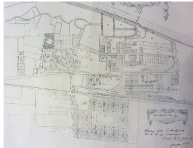
Plan de l'usine et de ses dépendances, 1/2500e, Georges Lisch architecte, 7 juin 1921 (AD Somme ; 49 Fi 2). Phot. Fournier Bertrand (reproduction) IVR22_20158006144NUCA
