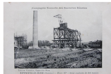
La grue roulante de 100 tonnes.
