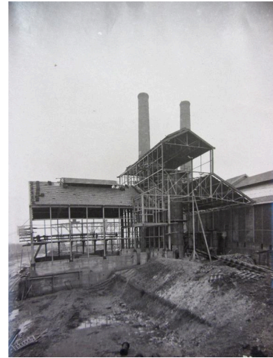
Vue extérieure du bâtiment principal et des cheminées de l'usine, 6 novembre 1922 (AD Somme ; 49 Fi 16).
