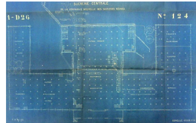
Plan détaillé de l'atelier principal de la sucrerie, 19 mai 1921 (AD Somme ; 5 M 623). Phot. Fournier Bertrand (reproduction) IVR22_20158006432NUCA
