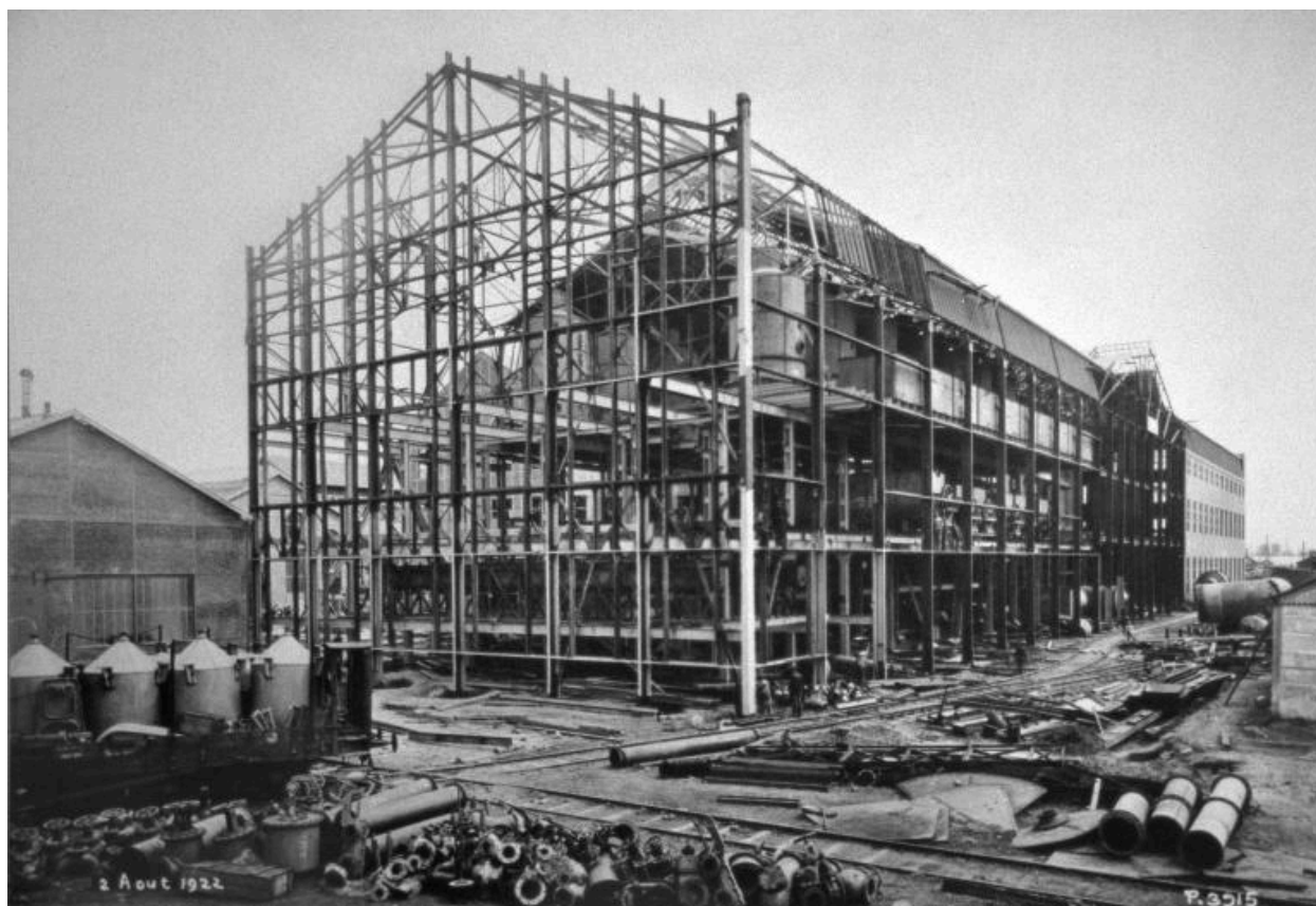
Structure métallique du grand atelier de fabrication, 2 août 1922 (Archives privées de l'entreprise).
