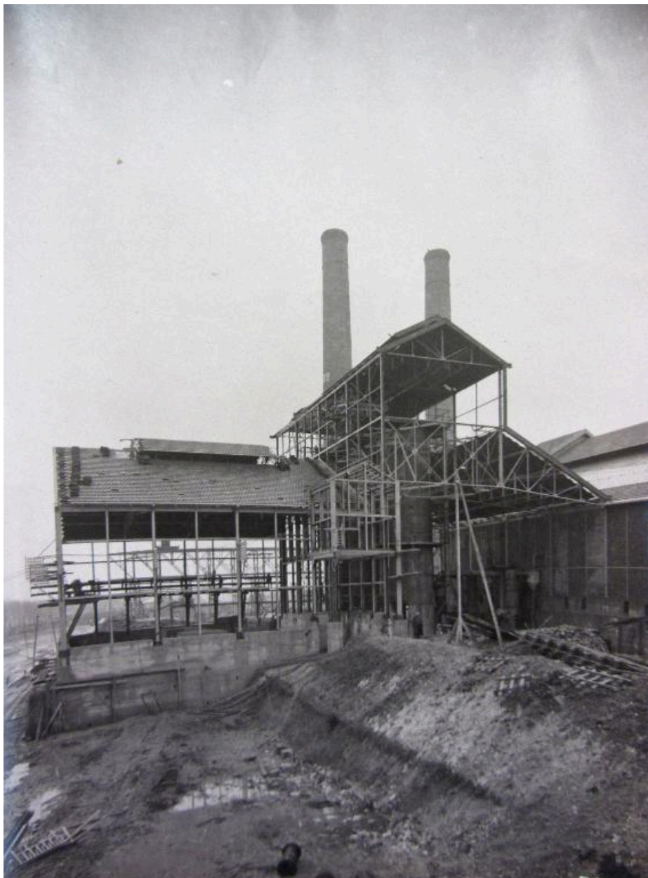
Vue extérieure du bâtiment principal et des cheminées de l'usine, 6 novembre 1922 (AD Somme ; 49 Fi 16).
