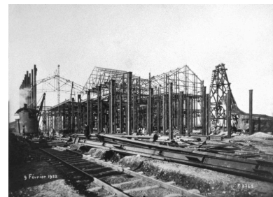
Montage de la structure métallique de la sucrerie, 9 février 1922 (Archives privées de l'entreprise). Phot. Bertrand Fournier IVR22_20008000406ZA
