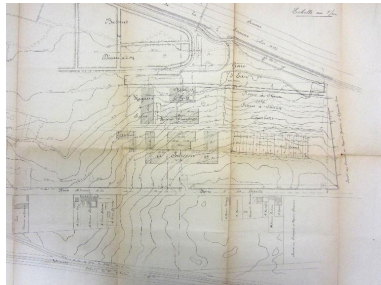
Plan d'ensemble de la sucrerie centrale d'Eppeville, avec indications des courbes de niveau, 1921. (AD Somme ; 5 M 624). Phot. Fournier Bertrand (reproduction) IVR22_20158006431NUCA
