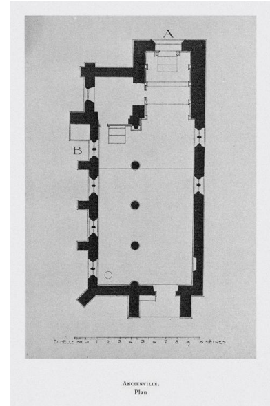
Plan de la précédente église, relevé par Étienne Moreau-Nélaton vers 1914 (Les Églises de chez nous. Arrondissement de Soissons, t. 1).
