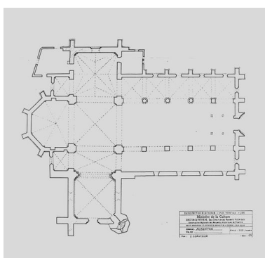
Plan de l'édifice, par Corvisier (CRMH). Phot. Thierry Lefébure IVR22_20020200383XB
