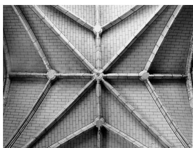
Transept sud : voûte nervurée appareillée comme la voûte à arrêtes triples. Phot. Franck Bürjes IVR22_19990201734X
