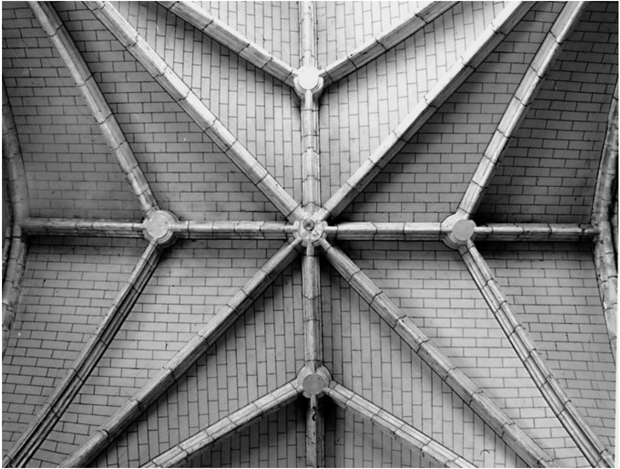
Transept sud : voûte nervurée appareillée comme la voûte à arrêtes triples.
