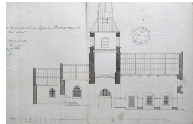
Coupe longitudinale de l'ancienne église en 1880 (AD Somme ; 99 O 1846).
