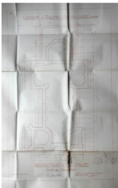
Plan des fondations, Louis Duthoit, avril 1928 (AD Somme ; 99 O 1846). Phot. Gilles-Henri Bailly (reproduction) IVR22_20158005272NUCA
