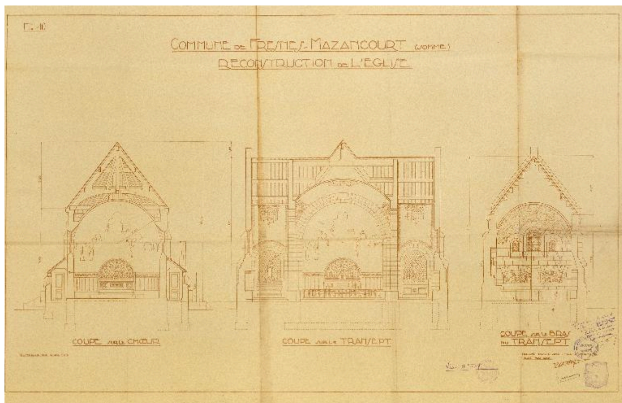
Coupes transversales, R. Duthoit (architecte), mai 1928 (AD Somme ; 99 O 1846).
