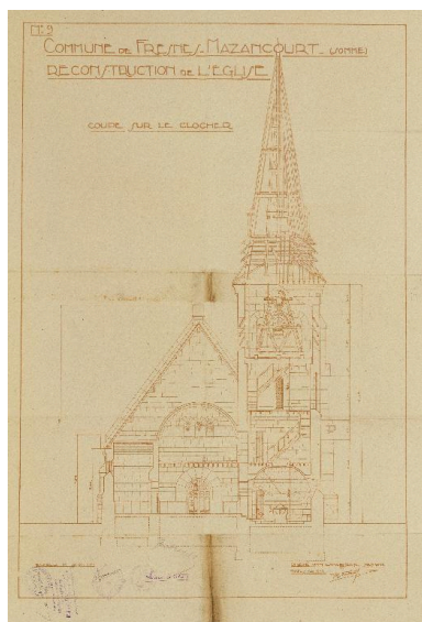
Fresnes-Mazencourt. Reconstruction de l'église, coupe sur le clocher.
