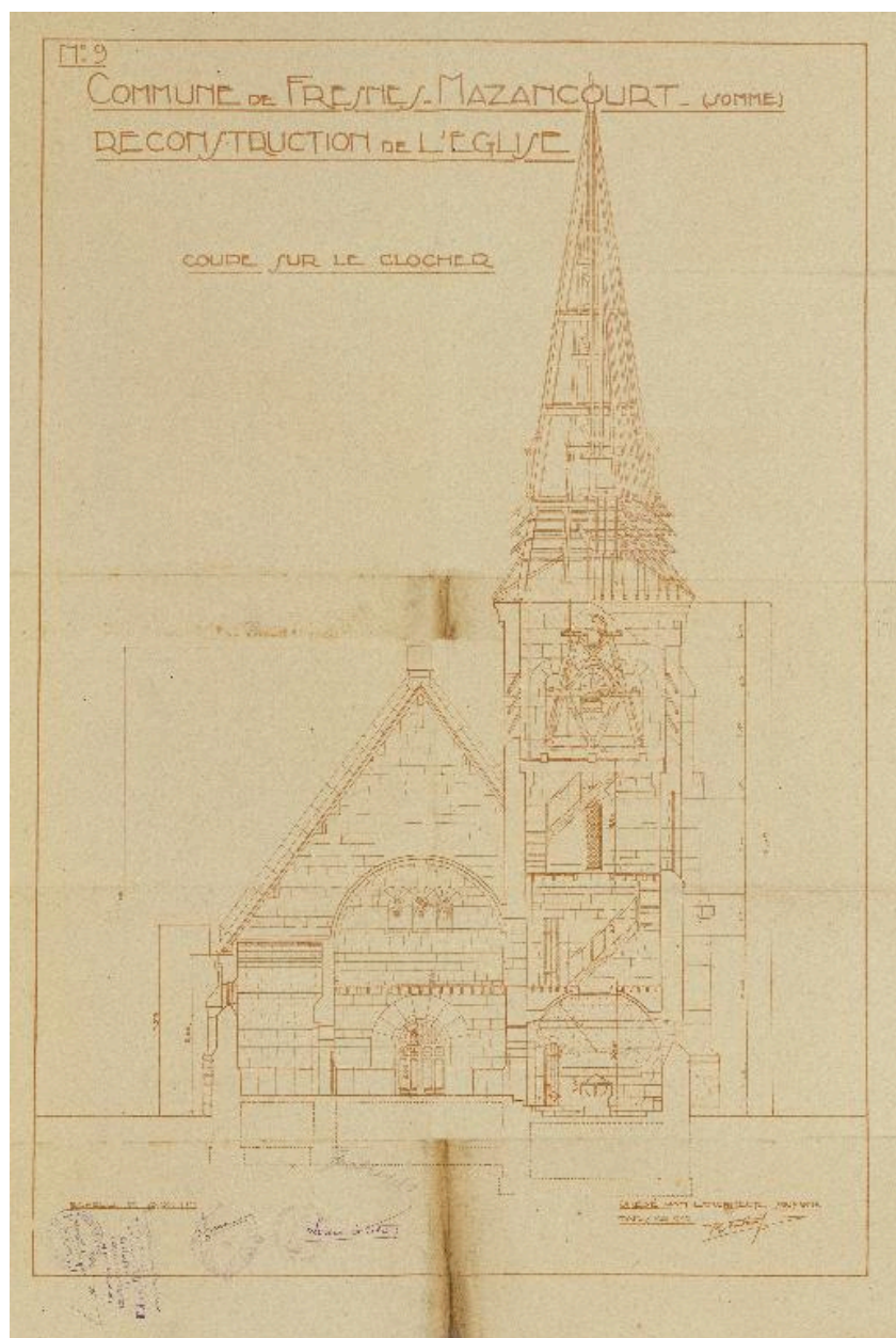
Fresnes-Mazencourt. Reconstruction de l'église, coupe sur le clocher. R. Duthoit (architecte), 1928 (AD Somme ; 99 O 1846).
