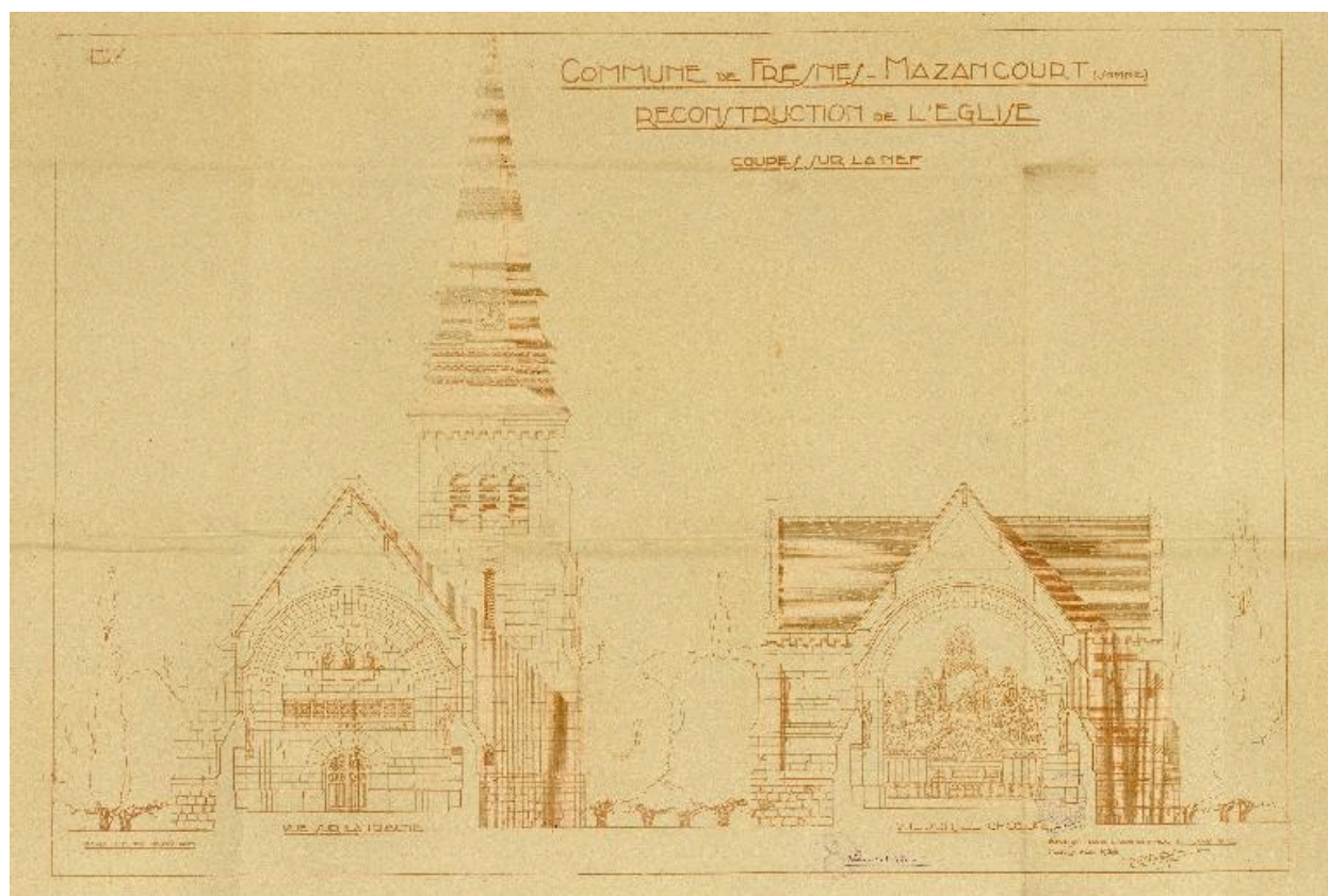
Coupes sur la nef, R. Duthoit (architecte), mai 1928 (AD Somme ; 99 O 1846).
