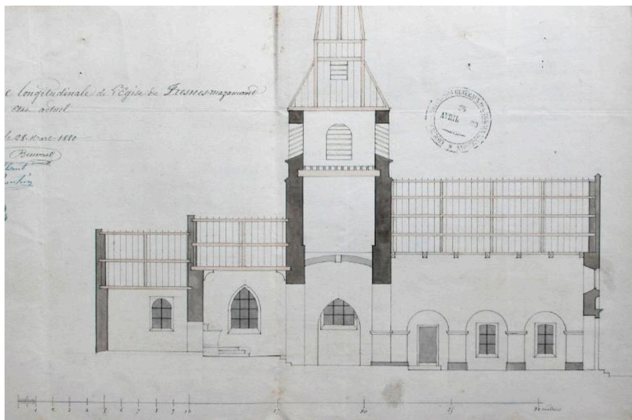
Coupe longitudinale de l'ancienne église en 1880 (AD Somme ; 99 O 1846).
