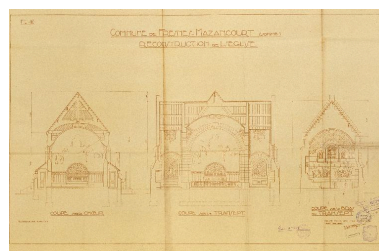
Coupes transversales, R. Duthoit (architecte), mai 1928 (AD Somme ; 99 O 1846). Phot. Thierry Lefébure IVR22_20068000515XAB
