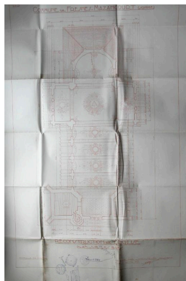
Plan sur les baies, Louis Duthoit architecte, avril 1928 (AD Somme ; 99 O 1846). Phot. Gilles-Henri Bailly (reproduction) IVR22_20158005273NUCA
