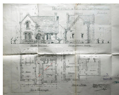
Plans et façades du presbytère, R. Duthoit (architecte), décembre 1929 (AD Somme ; 99 O 1846). Phot. Gilles-Henri Bailly (reproduction) IVR22_20158005280NUCA
