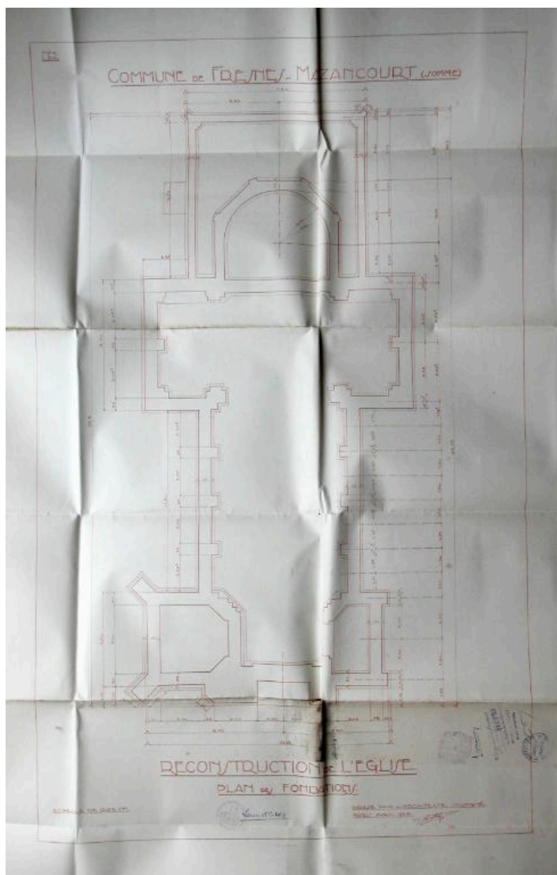
Plan des fondations, Louis Duthoit, avril 1928 (AD Somme ; 99 O 1846).
