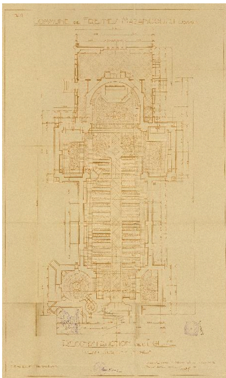
Fresnes-Mazencourt. Reconstruction de l'église, plan sur les niches. R. Duthoit (architecte), 1928 (AD Somme ; 99 O 1846).
