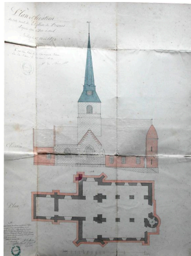
Plan et élévation nord de l'ancienne église, en 1874 (AD Somme ; 99 O 1846).
