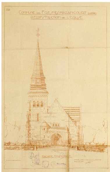
Elévation de la façade principale, R. Duthoit (architecte), mai 1928 (AD Somme ; 99 O 1846). Phot. Thierry Lefébure IVR22_20068000503XAB
