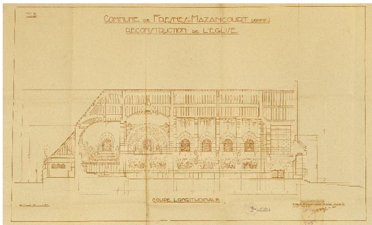
Coupe longitudinale, R. Duthoit (architecte), mai 1928 (AD Somme ; 99 O 1846).
