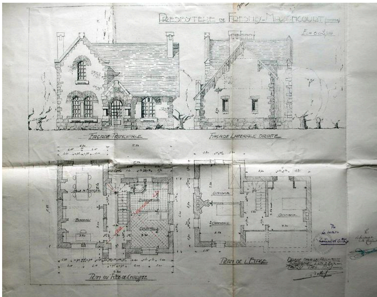
Plans et façades du presbytère, R. Duthoit (architecte), décembre 1929 (AD Somme ; 99 O 1846).
