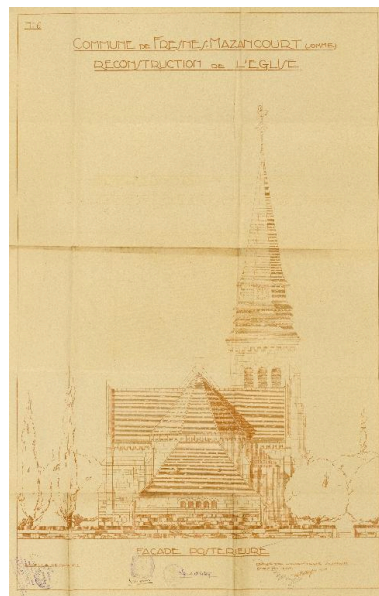
Elévation des façades postérieure, R. Duthoit (architecte), mai 1928 (AD Somme ; 99 O 1846). Phot. Thierry Lefébure IVR22_20068000505XAB
