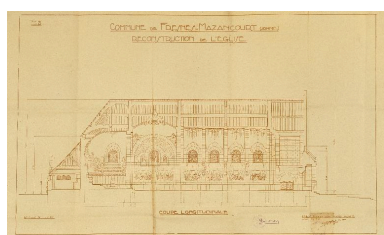
Coupe longitudinale, R. Duthoit (architecte), mai 1928 (AD Somme ; 99 O 1846). Phot. Thierry Lefébure IVR22_20068000511XAB
