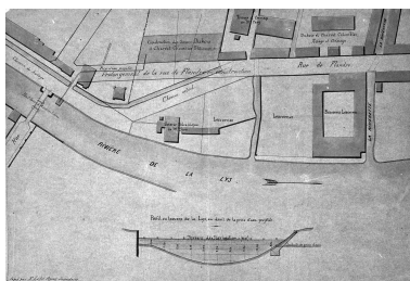
Duhem-Sion & Cie. Établissement d'une prise d'eau dans la Lys pour alimenter une machine à vapeur. Plan masse, 1869 (AD Nord ; S 3781). Repro. Philippe Dapvril IVR31_19875902582X
