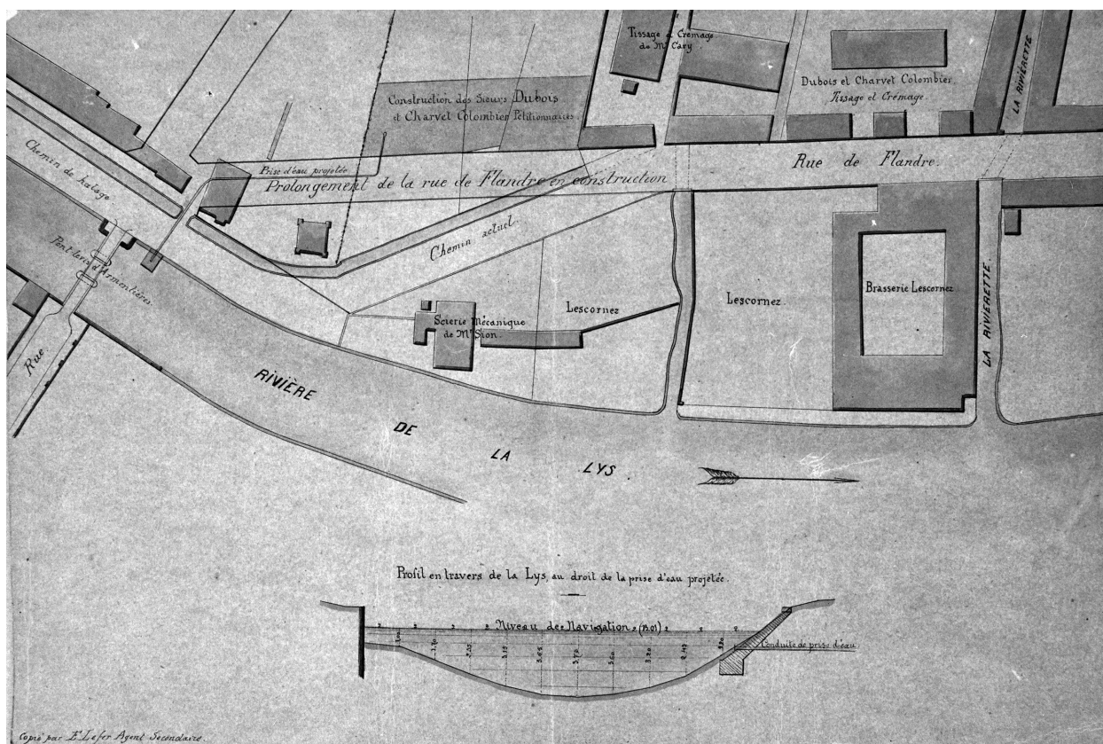
Duhem-Sion & Cie. Établissement d'une prise d'eau dans la Lys pour alimenter une machine à vapeur. Plan masse, 1869 (AD Nord ; S 3781).
