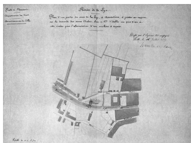
Duhem-Sion & Cie. Établissement d'une prise d'eau dans la Lys pour alimenter une machine à vapeur. Plan de situation, 1869 (AD Nord ; S 3781). Repro. Philippe Dapvril IVR31_19875902580X
