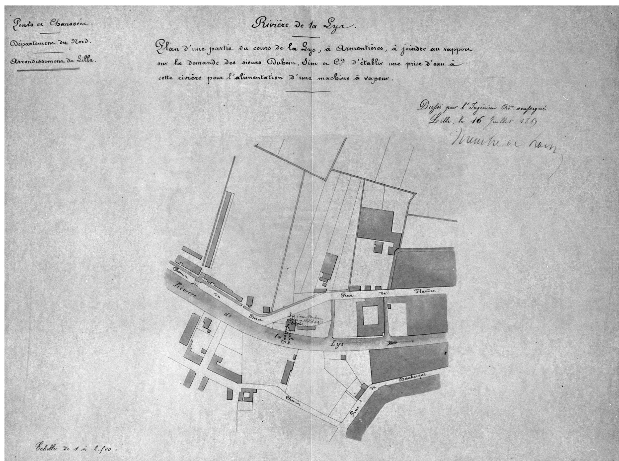
Duhem-Sion & Cie. Établissement d'une prise d'eau dans la Lys pour alimenter une machine à vapeur. Plan de situation, 1869 (AD Nord ; S 3781).
