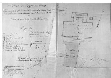
Autorisation demandée par Louis Sion d'installer une scierie mécanique. Plan masse, 1891 (AD Nord ; M 417620). Repro. Philippe Dapvril IVR31_19875902359X
