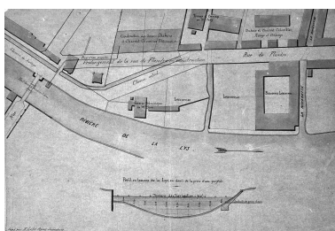
Duhem-Sion & Cie. Établissement d'une prise d'eau dans la Lys pour alimenter une machine à vapeur. Plan masse, 1869 (AD Nord ; S 3781). Repro. Philippe Dapvril IVR31_19875902582X
