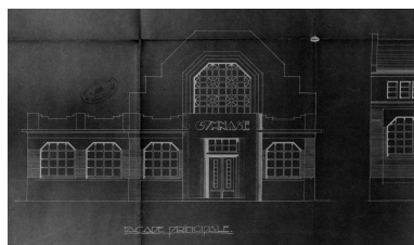
Projet de gymnase, élévation antérieure, plan, Adolphe Danis (architecte), [s.d.] (AD Nord ; O222/139). Repro. Thierry Petitberghien IVR31_20015902503X
