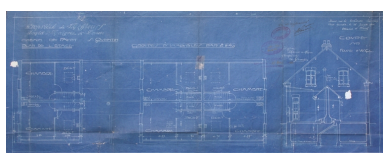
Plan des combles des logements construits à l'emplacement de la Cité Dambrun, par Mercier et Hivet, 1922 (AC Saint-Quentin).
