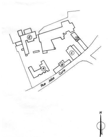
Schéma de situation : A. Logement patronal, B. Atelier, magasin, bureau, C. Atelier (four à recuire), D. Magasins, entrepôt, E. Grande fonderie. Dess. Monnehay-Vulliet Marie-Laure, Autr. Stéphane Gonet IVR32_20168000760NUD
