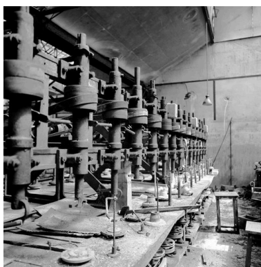
L'atelier de fabrication reconstruit après la guerre, banc de polissage. Phot. Patrick Glotain IVR22_19936000516X
