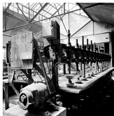
L'atelier de fabrication reconstruit après la guerre, banc de polissage. Phot. Patrick Glotain IVR22_19936000515X
