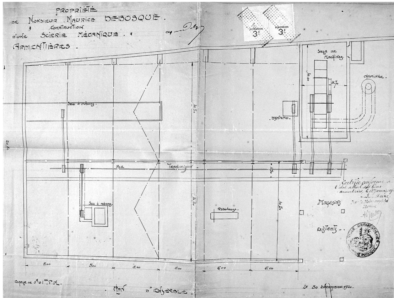
Maurice Debosque. Projet de construction d'une scierie mécanique. Plan masse, 1921 (AD Nord ; M 41710377).
