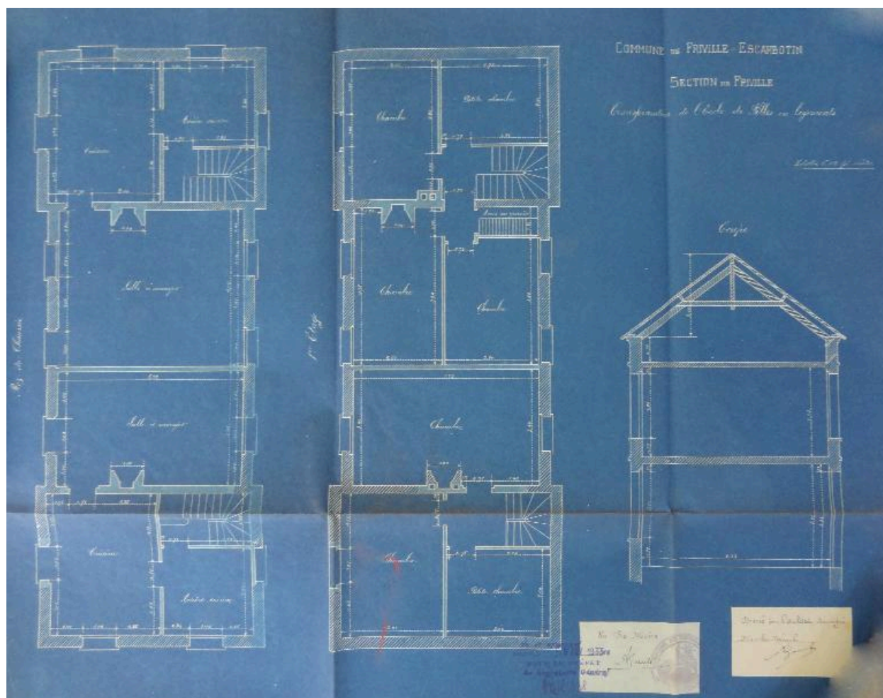
Plan de la réhabilitation de logements dans l'ancienne école des filles de Friville (AD Somme 99 O 1904).
