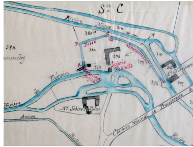
Plan d'ensemble des moulins de Troissereux et Fouquénie, extrait du plan cadastral, 1907. Phot. Fournier Bertrand (reproduction) IVR22_20046003017NUCA
