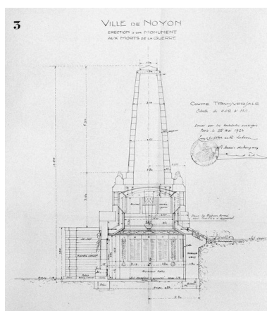
Coupe transversale, par E. Chifflet et R. Lefevre, 1924 (AD Oise ; série O). Phot. Jean-Michel Périn (reproduction) IVR22_19846000365XB
