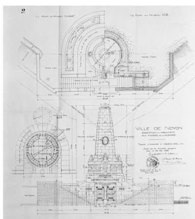
Plan du 2e niveau et élévation antérieure, par E. Chifflet et R. Lefevre, 1924 (AD Oise ; série O). Phot. Jean-Michel Périn (reproduction) IVR22_19846000364XB
