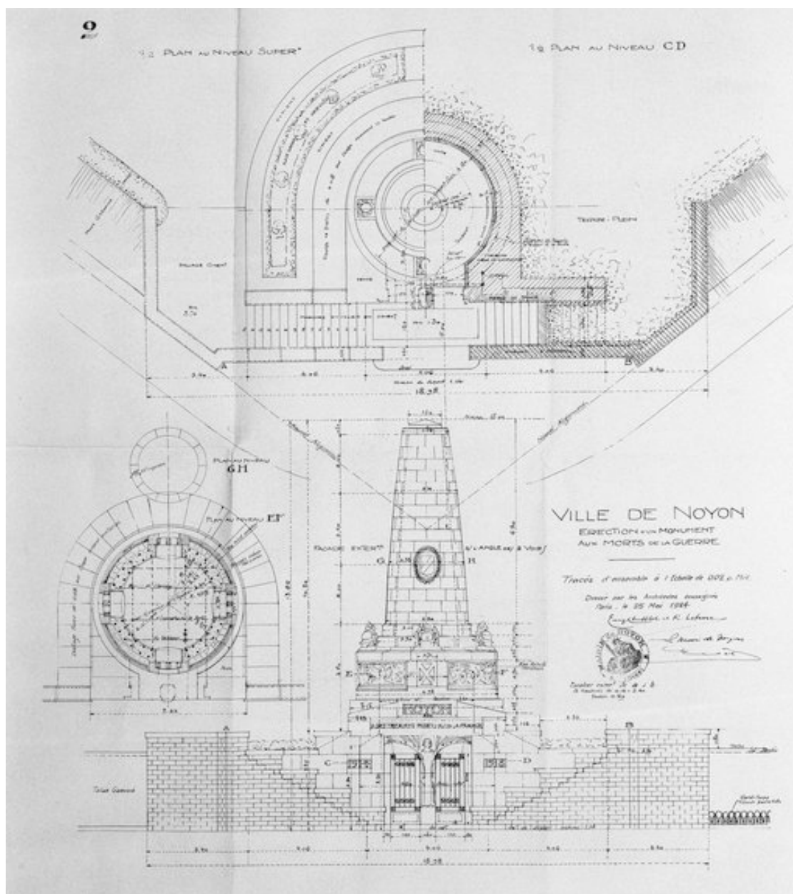
Plan du 2e niveau et élévation antérieure, par E. Chiffot et R. Lefevre, 1924 (AD Oise ; série O).
