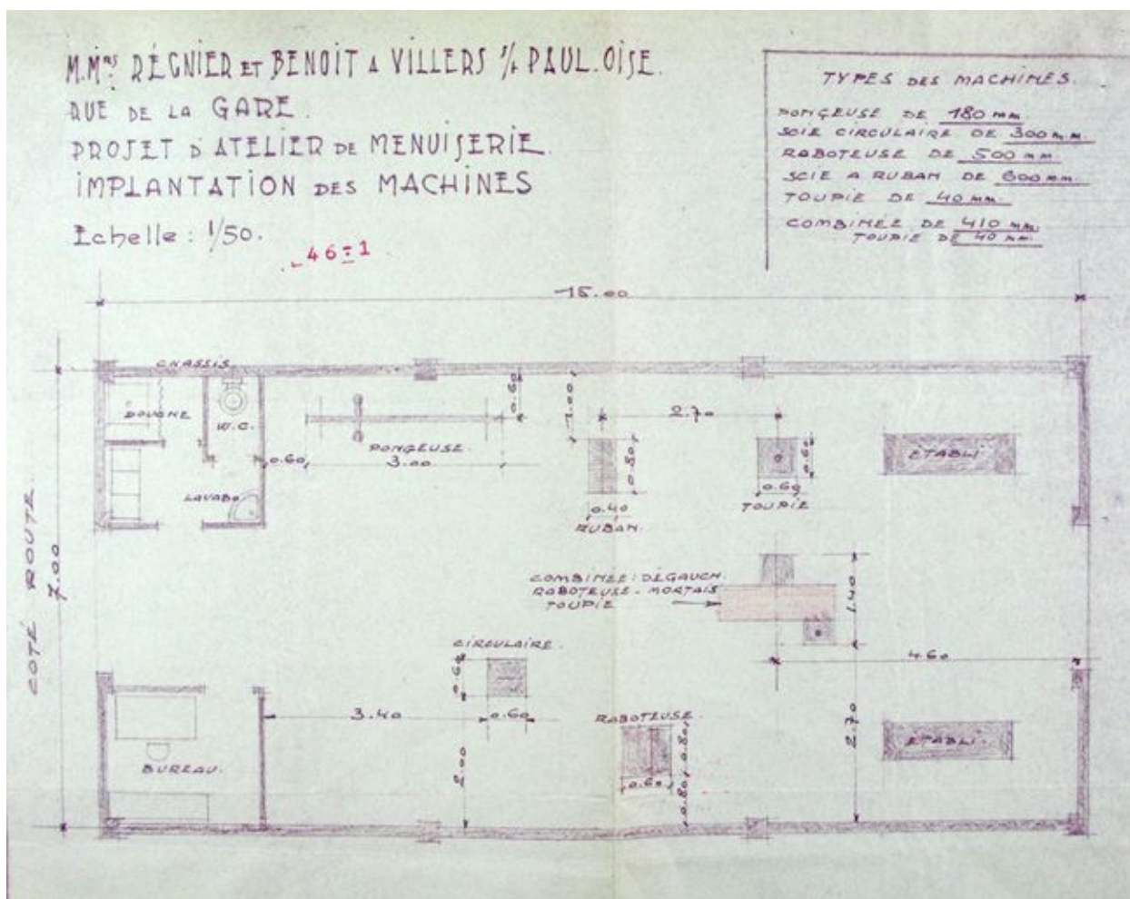
Plan de la menuiserie, 1959 (AD Oise ; 551W14467).
