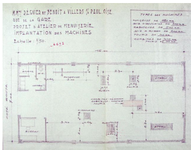
Plan de la menuiserie, 1959 (AD Oise ; 551W14467).
