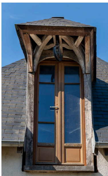
Lucarne avec poulie, n°2 rue de l'Église. Phot. Marc Kérignard IVR32_20226000822NUCA
