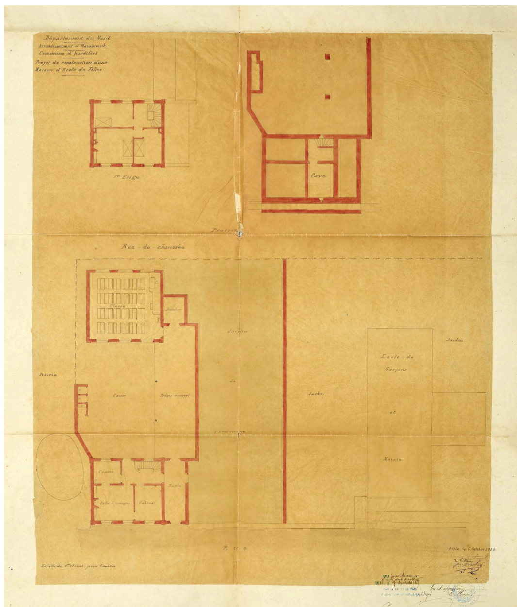
Projet de construction d'une maison d'école de filles - Plans. 1888 (AD Nord 2 O 276 / 18).
