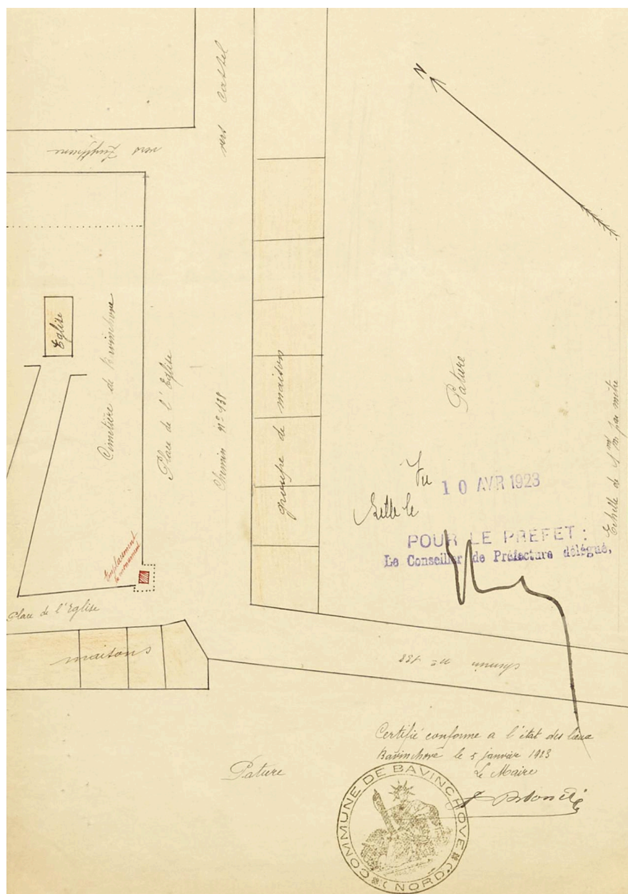
Plan de situation. Emplacement du monument aux morts, 1923 (AD Nord : 2 O 54/23).
