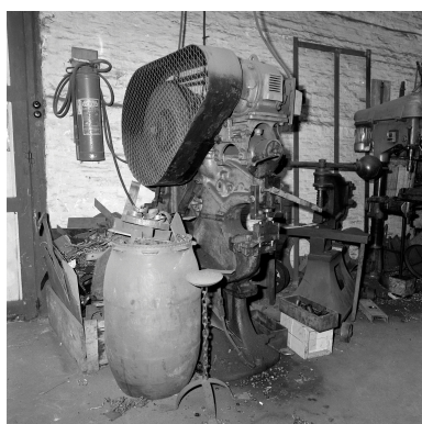
Atelier de fabrication, poinçonneuse (sans marque), vue gauche. Phot. Philippe Dapvril IVR31_19885900806X
