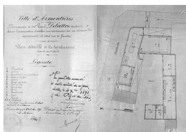
Demande d'installation d'une teinturerie déposée par Paul Delattre. Plan masse, 1891 (AD Nord ; M 417562). Repro. Philippe Dapvril IVR31_19875902397X
