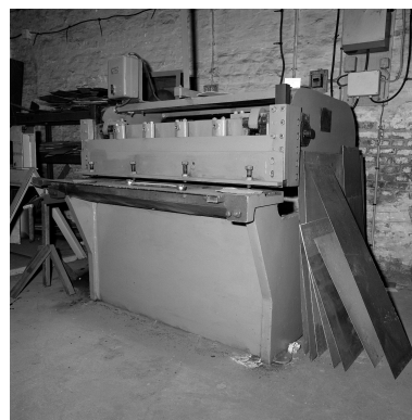
Atelier de fabrication, cisaille (sans marque). Phot. Philippe Dapvril IVR31_19885900813X
